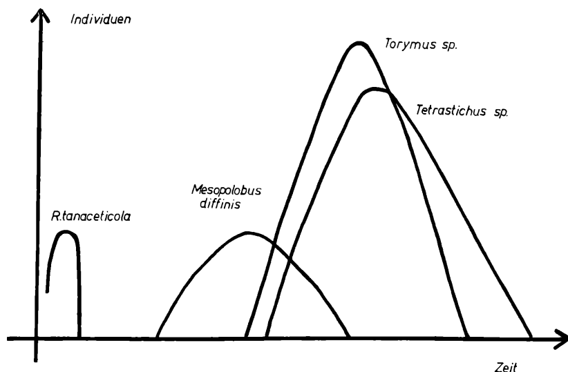
Abb. 3: Sukzession beim Schlüpfen der Parasiten von Rhopalomyia tanaceticola (KARSCH) im Frühjahr aus überwinterten Gallen (schematisch)
