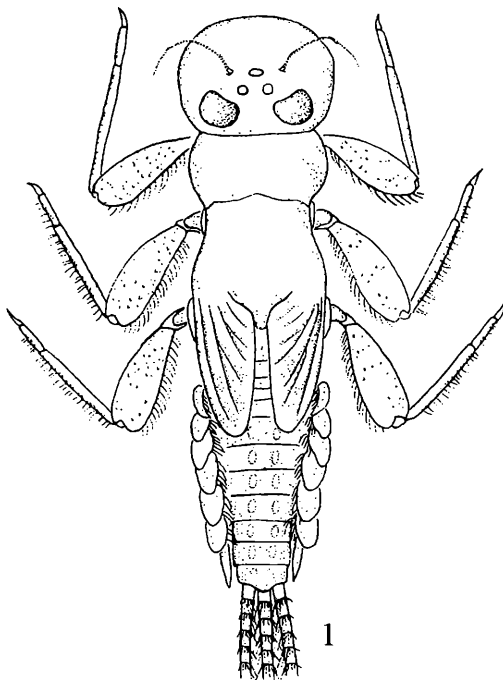
Abb. 1: Nympe von Parafronurus n. sp., Habitus.
