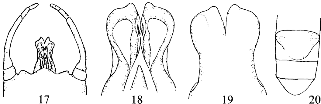
Abb. 17-20: Imagines, Genitalien von Parafronurus youi n. sp.: 17: Männchen, Genitalsegment, ventral; 18: Penis, ventral; 19: Penis, dorsal; 20: Weibchen, Genitalsegment, ventral.
