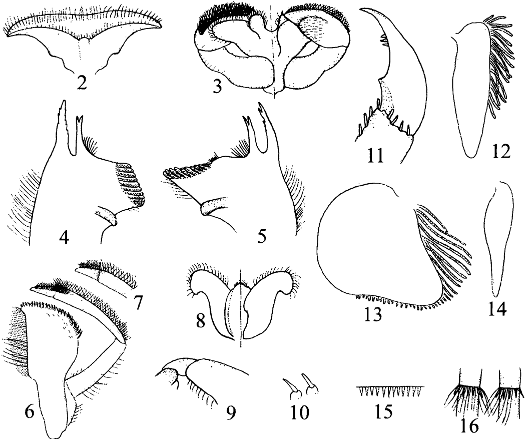
Abb. 2 – 16: Larvenmerkmale von Parafronurus n. sp. : 2: Labrum, ventral; 3: Labium, links ventral, rechts dorsal; 4: Mandibel, links; 5: Mandibel, rechts; 6: Maxille; 7: Maxillarpalpus, Apex; 8: Hypopharynx (links: dorsal; rechts ventral); 9: Hinterbein, Coxalregion; 10: Femurborsten; 11: Klaue; 12: Kieme I; 13: Kieme II; 14: Kieme VII; 15: Tergite: Hinterrandzacken, 16: Caudalfilamente: Dörnchenkränze und Haarbesatz an den Artikulationen.
