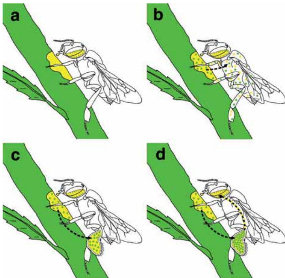
Abb. 5: Hypothetische Schritte der Evolution vom Duftmarkieren zum Parfümsammeln männlicher Prachtbienen. (a) Männlicher Vorfahr der Prachtbienen, der einen Zweig mit einem lipoiden Sekret aus der Labialdrüse (gelb) markiert. (b) Männlicher Vorfahr, der pflanzliche Düfte (grün), gelöst in sein eigenes Markierungssekret, angenommen hat. (c) Aktives Sammeln pflanzlicher Düfte mit Hilfe des lipoiden Sekrets in Hinterbeintaschen. (d) Anreicherung pflanzlichen Duftes in den Beintaschen durch Rückgewinnung des Labialdrüsensekrets. Verändert aus ELTZ et al. (2007).
