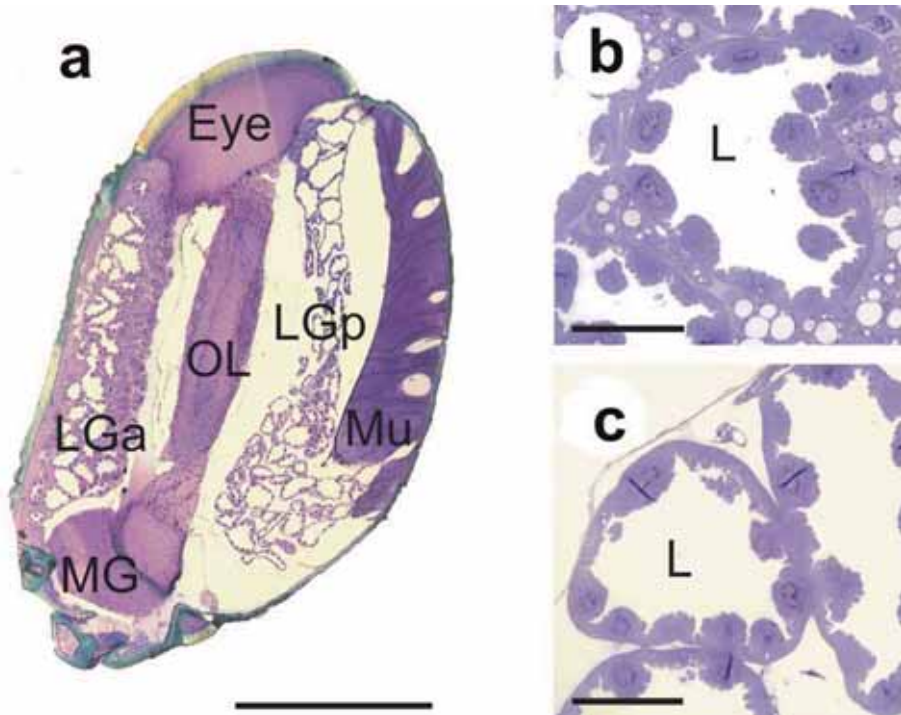
Abb. 2: Position und Struktur der kopfständigen Labialdrüsen eines Männchens von Euglossa viridissima . (a) Sagitaler Semidünnschnitt des Kopfes. Die Drüse nimmt einen großen Teil des Raumes um das Hirn ein und ist in einen vorderen Teil (LGa) unterhalb des Clypeus und einen hinteren Teil (LGp) hinter den Augen (Eye) und optischen Loben (OL) gegliedert. LGa (b) und LGp (c) sind aus Acini aufgebaut, die von einem einschichtigen Drüsenepithel gebildet werden, und im Falle des LGa von Fettkörperzellen umgeben sind. Größenskala ist 1mm in (a) und 50 \mu m in (b) und (c). MG=Mandibeldrüse, Mu=Muskel; verändert aus ELTZ et al. (2007).
