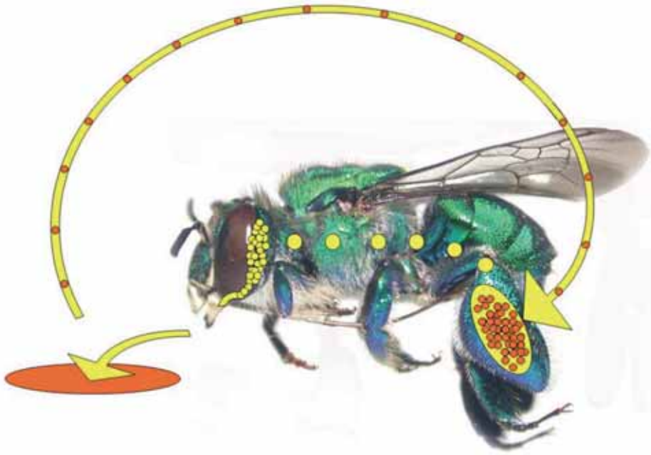
Abb. 4: Parfum-anreicherung. Das schwerflüchtige Labialdrüsensekret (gelb) wird auf die duftende Oberfläche gesputet, die flüchtigen Duftstoffe (orange) lösen sich darin und werden schließlich zusammen mit dem Sekret in die Hinterbeintaschen transferiert. Im weiteren Verlauf wird der Großteil des Sekrets wieder aus den Beintaschen sequestriert und über die Hämolymphe zurück in die Labialdrüsen transportiert, wo es für weitere Sammelvorgänge zur Verfügung steht. In den Hinterbeintaschen reichert sich in Folge ein immer konzentrierteres Parfum aus exogenen Komponenten an.
