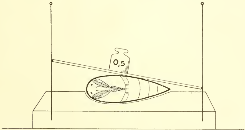
Abb. 94. Versuchsanordnung.
