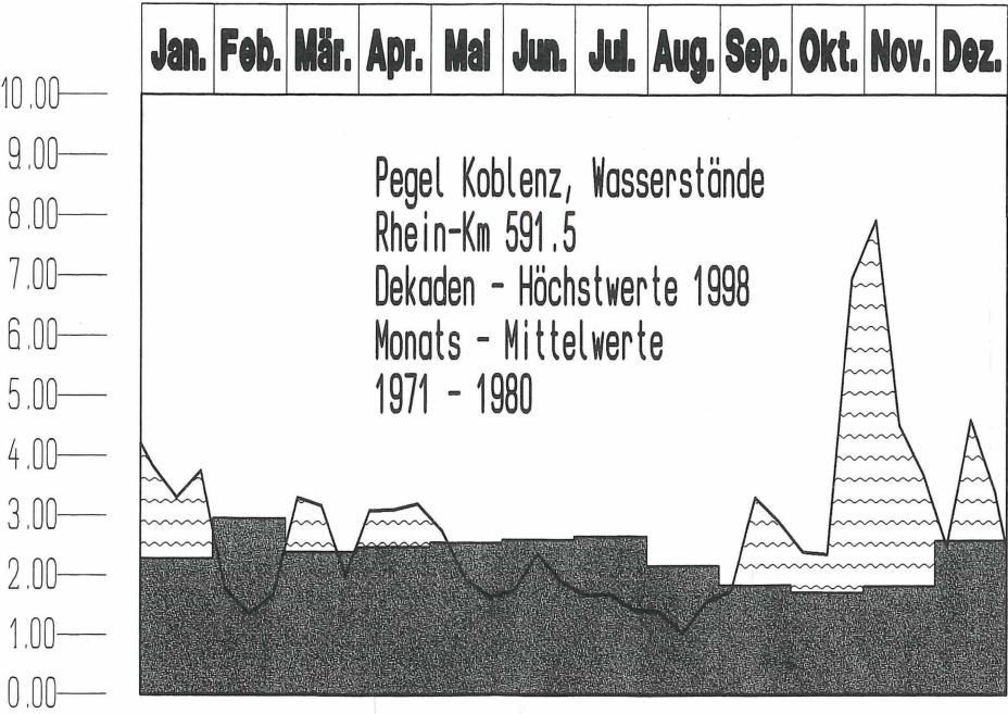
Wasserstände des Rheins (Pegel Koblenz bei Fluss-km 591,5) mit Dekaden-Höchstwerten 1998 und dem längjährigen Monats-Mittelwerten (1971-1980).
