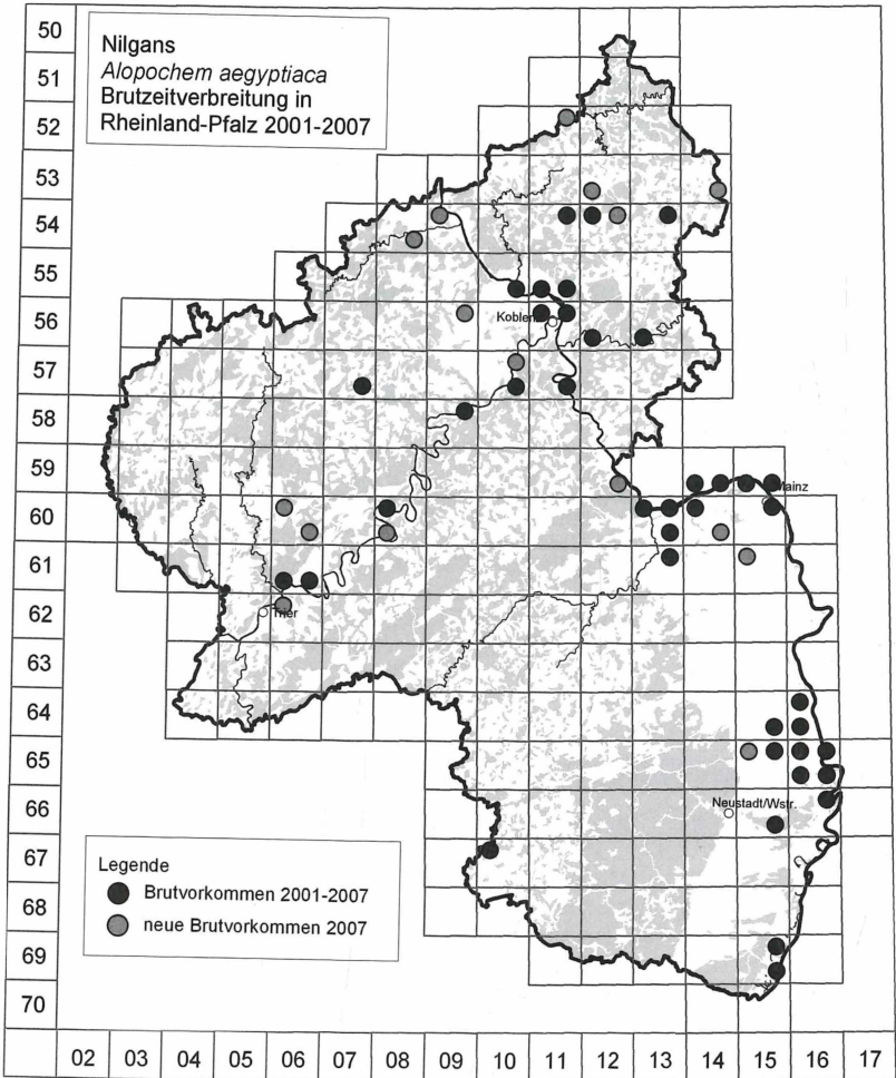
Abb. 7: Brutverbreitung der Nilgans ( Alopochen aegyptiaca ) in Rheinland-Pfalz 2001-2007 (besetzte TK25-Quadranten).
