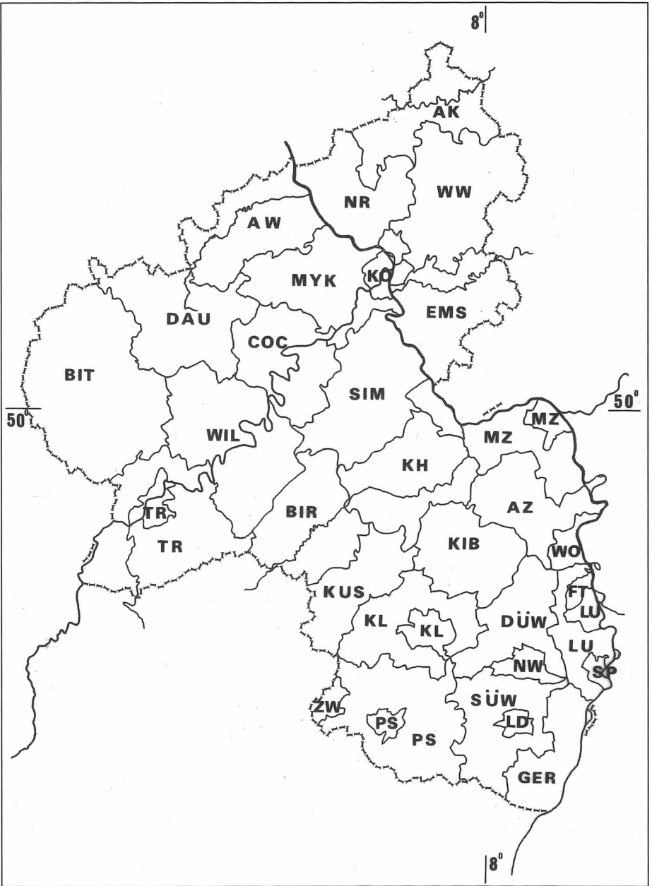
Abb. 2: Grenzen der Landkreise und Kreisfreien Städte in Rheinland-Pfalz (aus KUNZ & SIMON 1987). Der Rhein-Pfalz-Kreis wird jetzt mit RP statt LU abgekürzt, d. h. LU ist nun beschränkt auf die Stadt Ludwigshafen.
