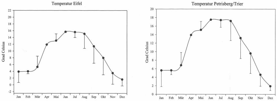
Abb. 5: Monatsmittelwerte der Temperatur an zwei verschiedenen Stationen in Rheinland-Pfalz 2007. Die Fehlerbalken geben die Abweichung vom langjährigen Mittel der letzten 30 Jahre an. [Quelle: DWD.]
