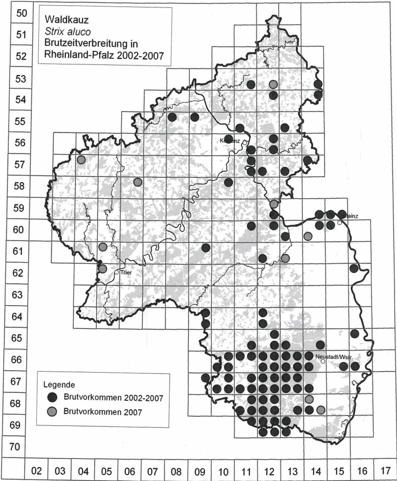
Abb. 15: Brutzeitverbreitung des Waldkauzes ( Strix aluco ) in Rheinland-Pfalz 2001-2007 (besetzte TK25-Quadranten).
