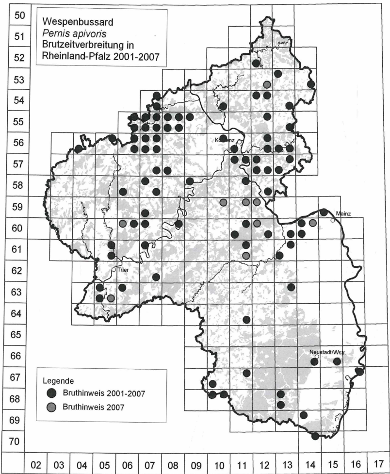
Abb. 11: Brutzeitverbreitung des Wespenbussards ( Pernis apivorus ) in Rheinland-Pfalz 2001-2007 (besetzte TK25-Quadranten).
