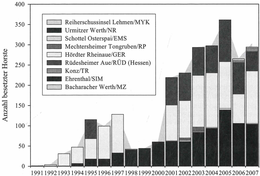
Abb. 9: Brutbestand des Kormorans ( Phalacrocorax carbo ) in Rheinland-Pfalz 1991-2007 für die einzelnen Kolonien. Die Gesamthöhe der Säulen entspricht dem rheinland-pfälzischen Brutbestand inklusive der Kolonie auf hessischer Seite.
