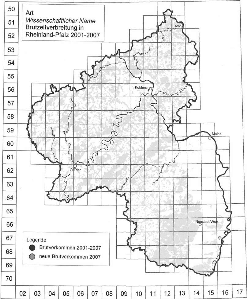
Abb. 1: Kartengrundlage zur Darstellung der Verbreitung auf TK25-Quadranten-Basis. Bewaldete Flächen sind grau hinterlegt.
