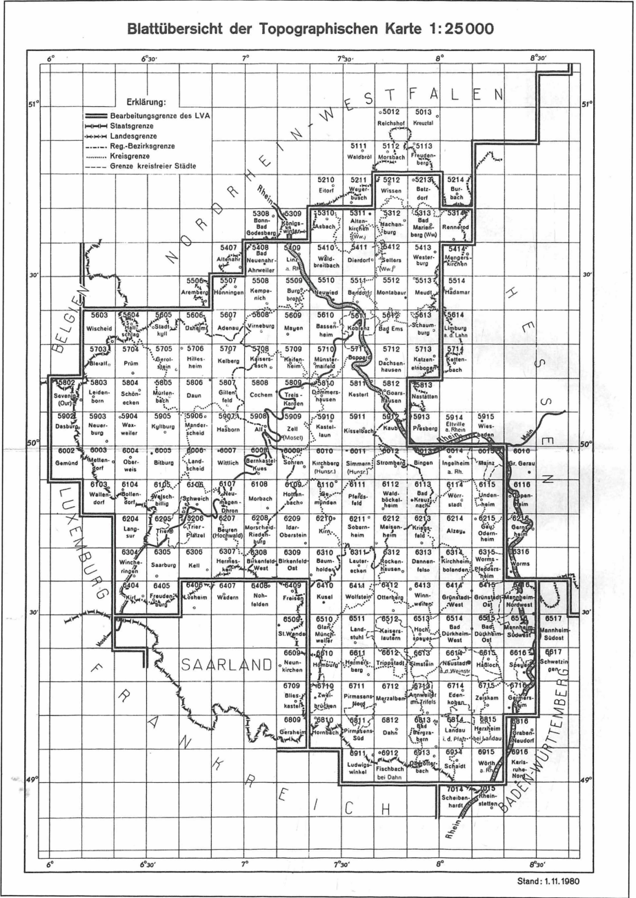
Abb. 4: Blattübersicht der Topographischen Karten 1:25.000 für Rheinland-Pfalz (Landesamt für Vermessung und Geobasisinformation Rheinland-Pfalz).
