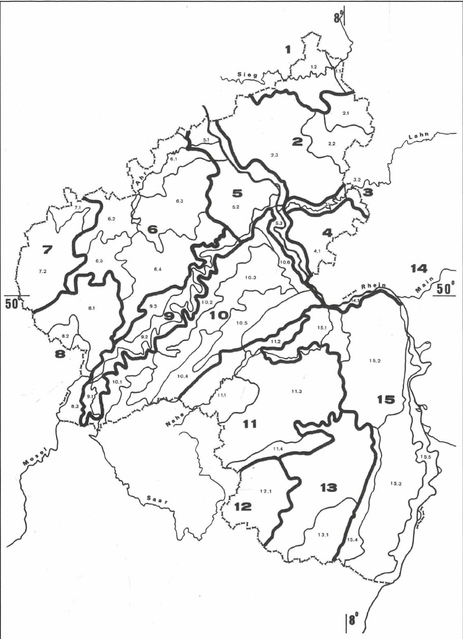
Abb. 3: Naturräumliche Gliederung von Rheinland-Pfalz (aus KUNZ & SIMON 1987). Erläuterung s. Text S. 13.
