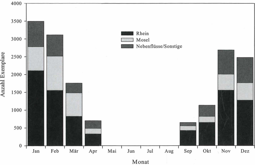
Abb. 10: Ergebnis der Kormoranschlafplatz-Synchronzählungen in Rheinland-Pfalz 2007 an 44 Schlafplätzen. N = 16.033 Ex. Die Gesamthöhe der Säulen gibt den Gesamtbestand wieder.
