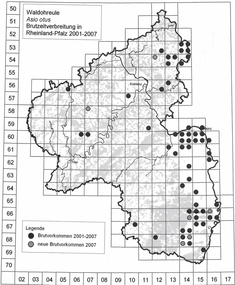
Abb. 14: Brutzeitverbreitung der Waldohreule ( Asio otus ) in Rheinland-Pfalz 2001-2007 (besetzte TK25-Quadranten).
