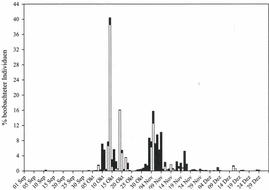
Abb. 12: Zeitlicher Verlauf des Kranich ( Grus grus ) – Durchzuges in Rheinland-Pfalz 2001-2006 (schwarz) und 2007 (grau). Prozentanteil täglich beobachteter Individuen an der Gesamtheit aller Individuen im Frühjahr (vorherige Seite, n = 446.980 Ex.) und Herbst (diese Seite, n = 325.143 Ex.).
