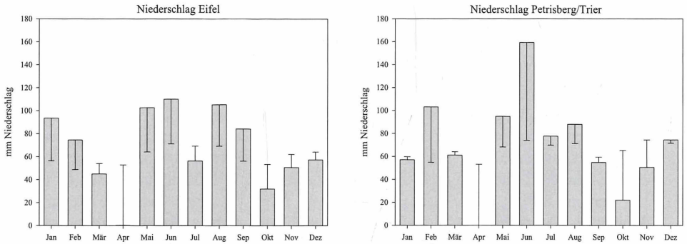
Abb. 6: Monatliche Niederschlagssummen an zwei verschiedenen Stationen in Rheinland-Pfalz 2007. Die Fehlerbalken geben die Abweichung vom langjährigen Mittel der letzten 30 Jahre an. [Quelle: DWD.]
