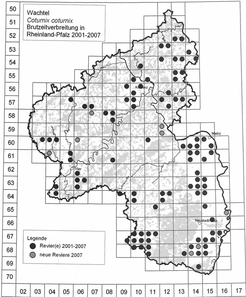
Abb. 8: Brutzeitverbreitung der Wachtel ( Coturnix coturnix ) in Rheinland-Pfalz 2001-2007 (besetzte TK25-Quadranten).
