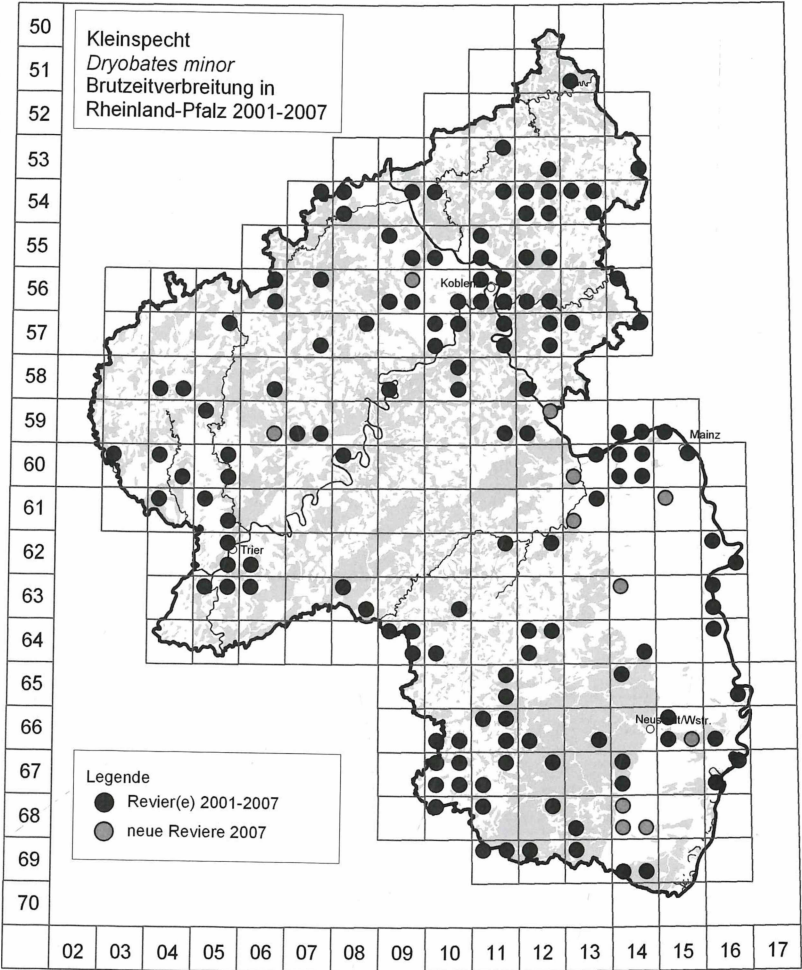
Abb. 17: Brutzeitverbreitung des Kleinspechts ( Dryobates minor ) in Rheinland-Pfalz 2001-2007 (besetzte TK25-Quadranten).
