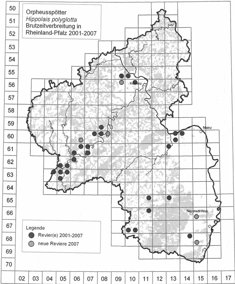
Abb. 18: Brutzeitverbreitung des Orpheusspötters ( Hippolais polyglotta ) in Rheinland-Pfalz 2001-2007 (besetzte TK25-Quadranten).
