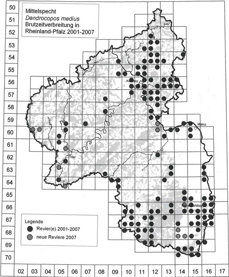
Abb. 16: Brutzeitverbreitung des Mittelspechts ( Dendrocopos medius ) in Rheinland-Pfalz 2001-2007 (besetzte TK25-Quadranten).
