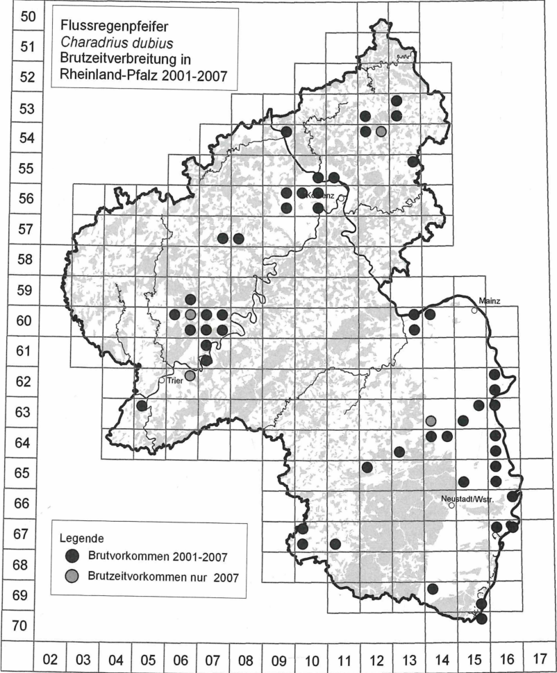
Abb. 13: Brutzeitverbreitung des Flussregenpfeifers ( Charadrius dubius ) in Rheinland-Pfalz 2001-2007 (besetzte TK25-Quadranten).
