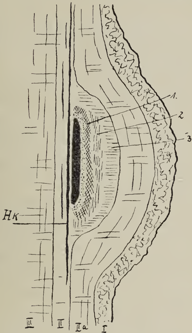
Fig. 5. Harzgalle im Stammlängsschnitt (schematisch). Bezeichnung wie in Fig. 4.
