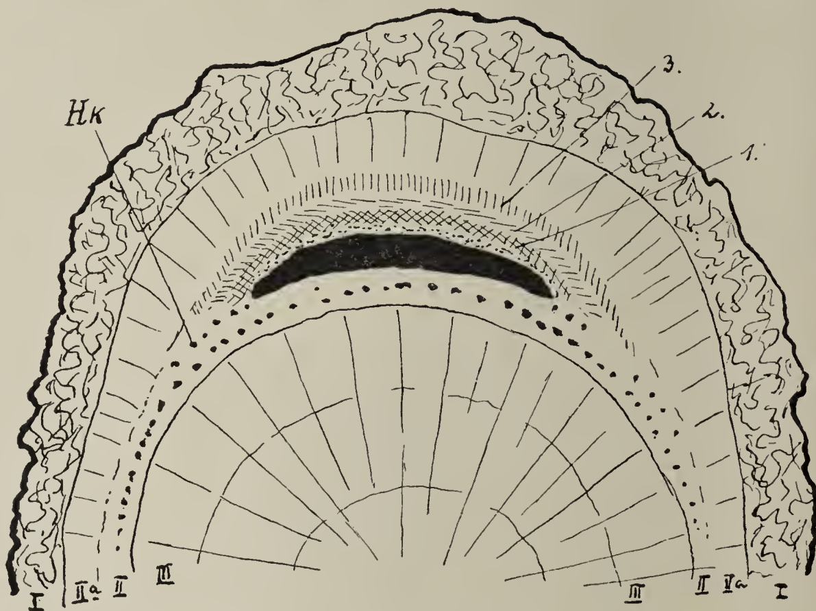
Fig. 4. Harzgalle im Stammquerschnitt (schematisch). Bezeichnung wie in Fig. 1. 1—3 die drei Randschichten der Harzgalle. 1. Tracheidalparenchym, das später der Verharzung anheimfällt; 2. Tracheidalparenchym, dessen Zellen zwar noch Harz führen, aber nicht zugrunde gehen; 3. harzfreie Randschicht des Tracheidalparenchyms.
