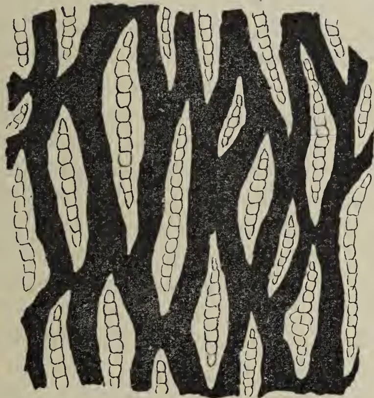
Fig. 3. Harzfluss. Tangentialschnitt durch die Harzkanalschicht, die Kanalanastomosen zwischen den Markstrahlen zeigend.
