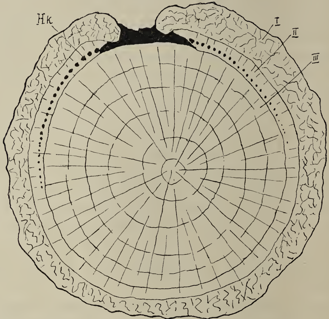
Fig. 1. Schematische Darstellung der Entstehung des Harzflusses am Stammquerschnitt. I Rinde. II Nach der Verwundung entstandenes Neuholz mit Harzkanälen (HK) in der Umgebung der Wunde. III Altholz. Das Harz ist schwarz gehalten.
