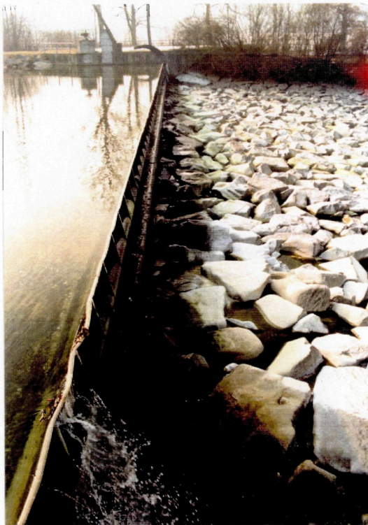
Abb. 130: Das Stegmühlwehr
