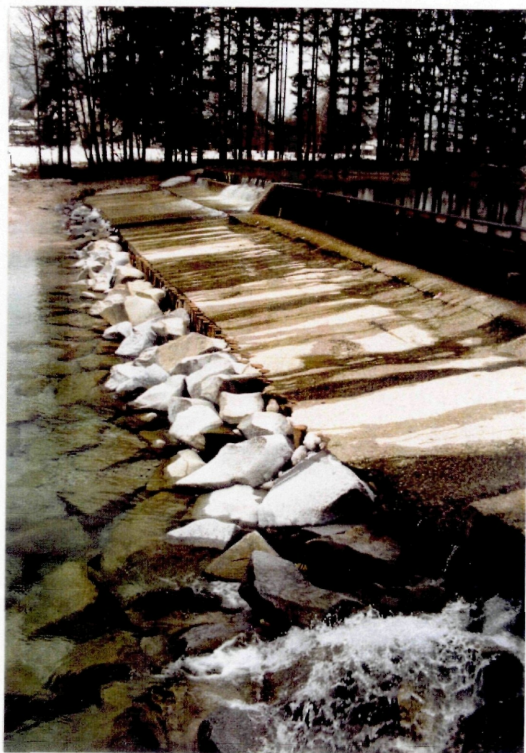
Abb. 68: Unterwasserseitig ist das Wehr durch vorgelagerte Granitsteine gesichert
