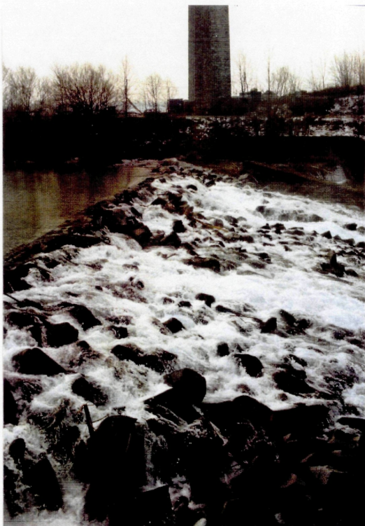
Abb. 124: Die 6 m Höhendifferenz werden über eine Granitsteinrampe überwunden
