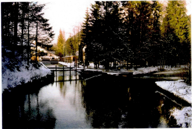
Abb. 3: Wehranlage des Habernauerwehres, links der Sagbach mit dem Rechenbauwerk vor dem Turbinenhaus der Habernauersäge.
