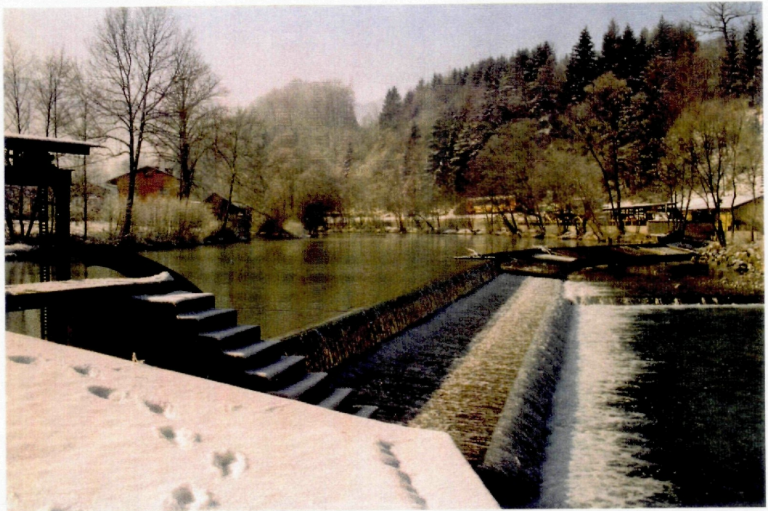
Abb. 49: das Sagbauernwehr
