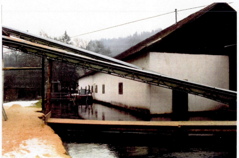
Abb. 111: Rechenbauwerk und Einlauf in die Sattelmühle
