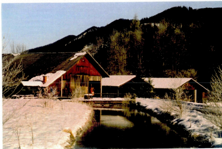
Abb. 10: Blick über einen Teil des 177 m langen Oberwasserkanals zum Krafthaus
