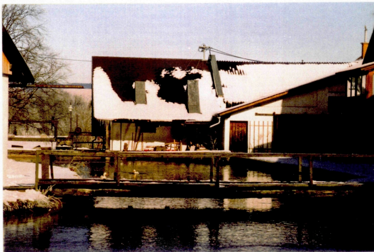
Abb. 40: Steg über den Mühlbach, das Rechenbauwerk und Blick auf das Krafthaus der Redlmühle
