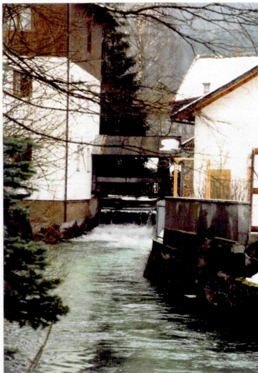
Abb. 38: Auslauf des E-Werkes II. Aufgrund der engen Verbauung im Ortszentrum von Grünau sind die Uferböschungen mit Steinen aufgemauert. Teilweise schließen sich Gärten aber auch Wohnhäuser an.
