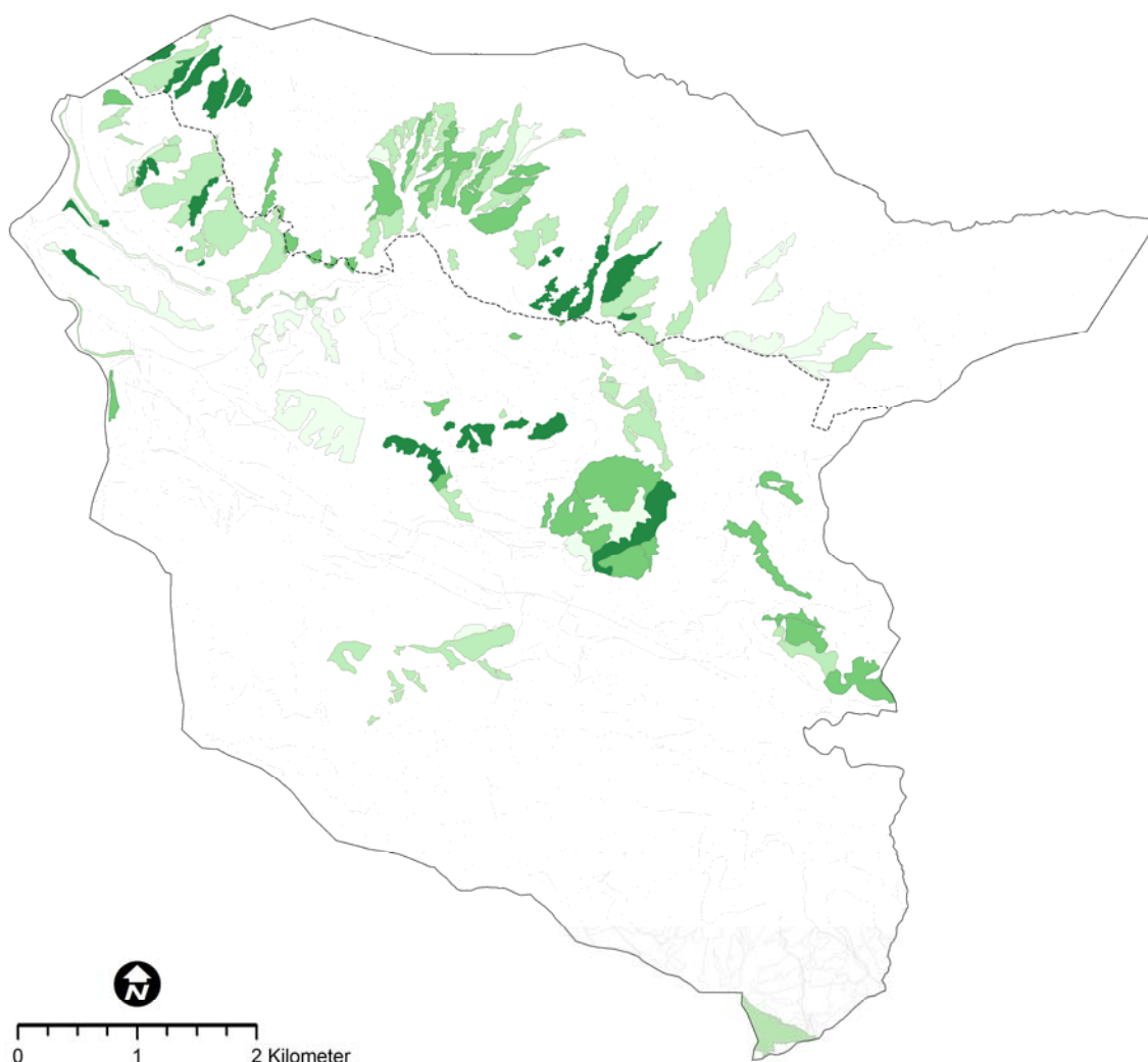
Karte 12: Schneeheide-Kiefernwälder (5.20.1)
