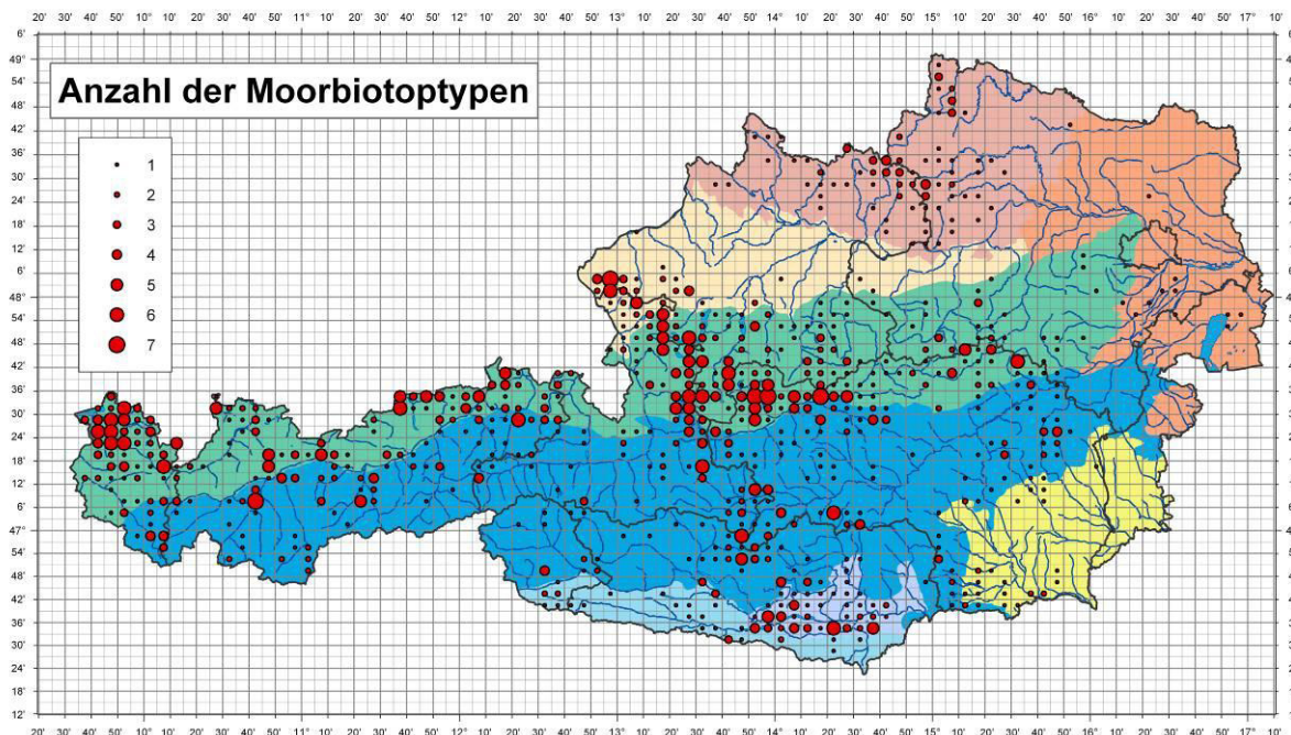
Abb. 3: Raster-Summenkarte der heutigen Verbreitung der 10 Moorbiototypen Österreichs (Quelle: Datenbank der Biotypen Österreichs, Umweltbundesamt, 2009). Entwässerte oder zerstörte Moorflächen sind hier nicht ausgewiesen.
