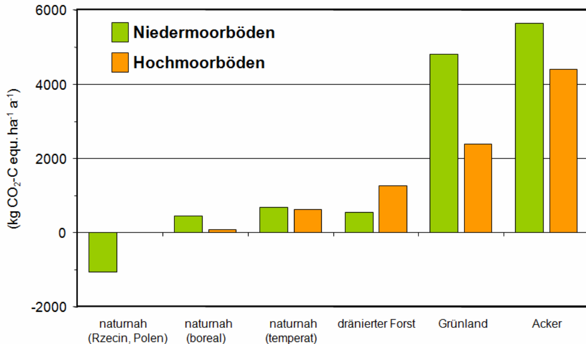
Abb. 2: Durchschnittlicher CO 2 Ausstoß aus Böden naturnaher Moore und unterschiedlich intensiv genutzter ehemaliger Moore 7
