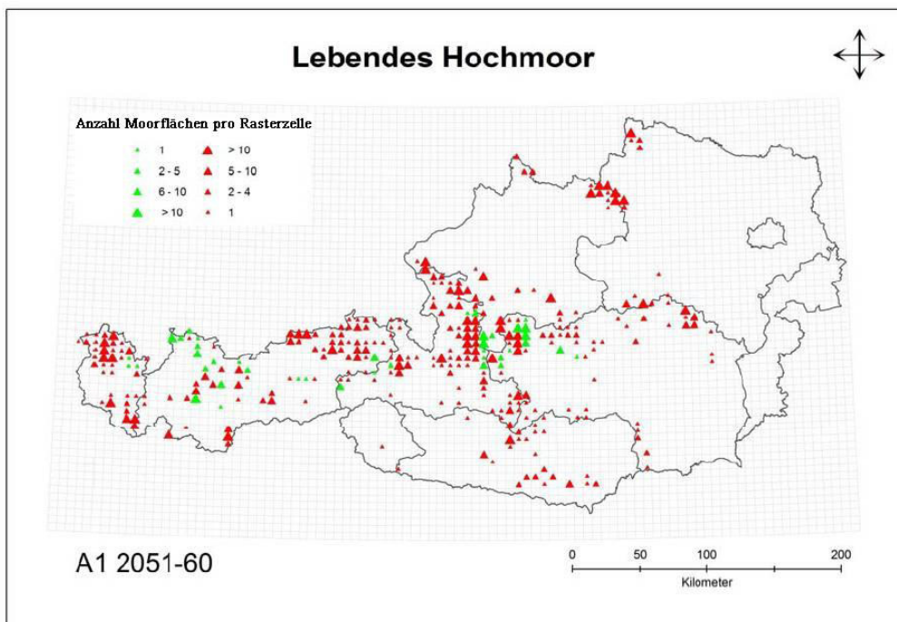
Abb. 5. Klimatische Gefährdungssituation der Vorkommen des Biotoptyps „Lebendes Hochmoor“ unter dem Klimawandelszenario A1 in der Mitte des 21. Jahrhunderts bei einem Temperaturanstieg von etwa 2,3 °C. Rote Dreiecke symbolisieren Moore, die einem hohen klimatischen Risiko ausgesetzt sind, grüne Dreiecke solche, die einem geringen klimatischen Risiko ausgesetzt sind. Je größer die Symbole, desto mehr Hochmoorflächen befinden sich in der Rasterzelle.
