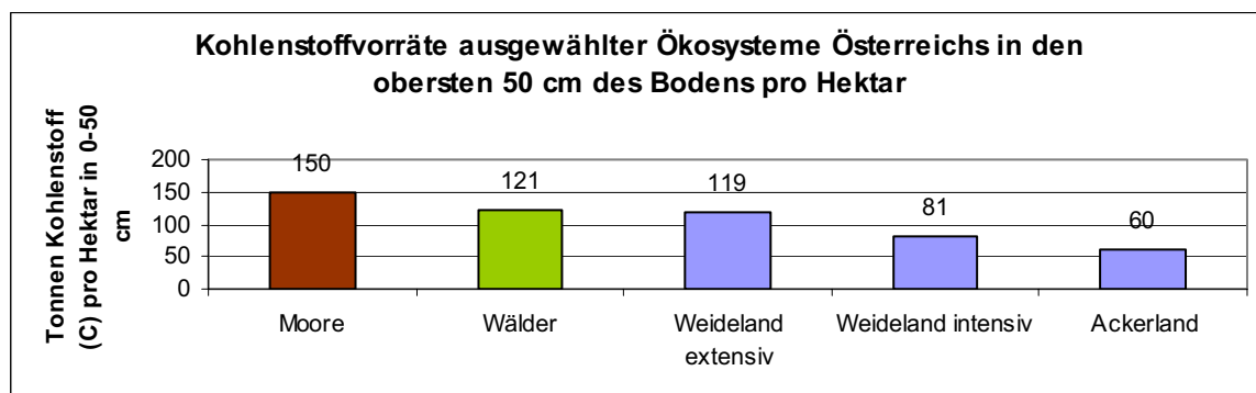
Abb. 1.: Kohlenstoffvorräte in den obersten 50 cm des Bodens ausgewählter Ökosysteme gemäß Nationaler Treibhausgasinventur NIR 2009, eigene Darstellung
