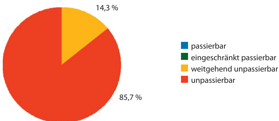
Abb. 49: Passierbarkeit der Querbauwerke für abwärtswandernde Fische im Steinerbach.
