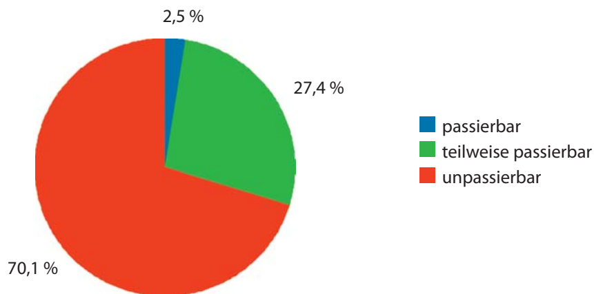
Abb. 17: Passierbarkeit der Querbauwerke für Benthosorganismen im Irr- und Mondsee-System.
