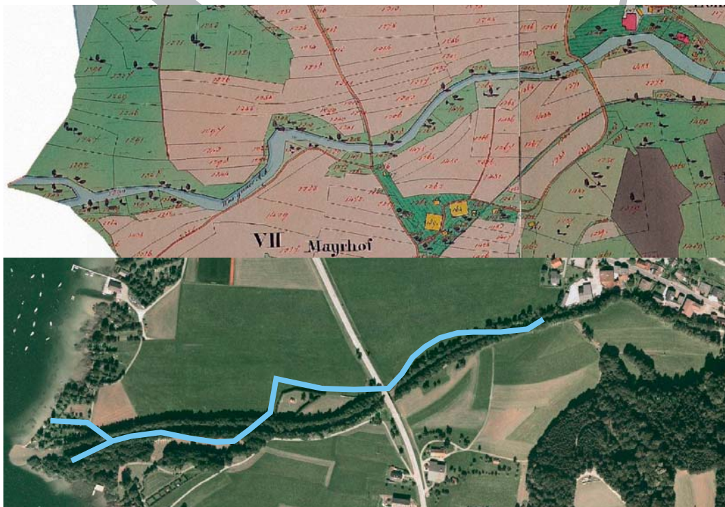
Abb. 134: Ab der Ortschaft Loibichl wurde der Lauf der Wangauer Ache begradigt (blaue Linie: alter Lauf) und durch Ufer- und Sohlsicherungen fixiert. Uferdämme sollen Überschwemmungen vorbeugen (oben Franziszeischer Kataster (Franziszeische Landesaufnahme von 1824, © Land Oberösterreich, Original: Oö Landesarchiv), unten Google Maps).
