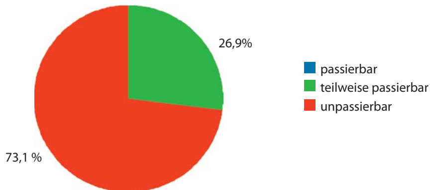
Abb. 33: Passierbarkeit der Querbauwerke für Benthosorganismen im Pangraben.
