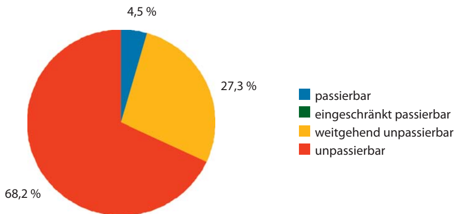
Abb. 60: Passierbarkeit der Querbauwerke für aufwandernde Fische in der Wangauer Ache.
