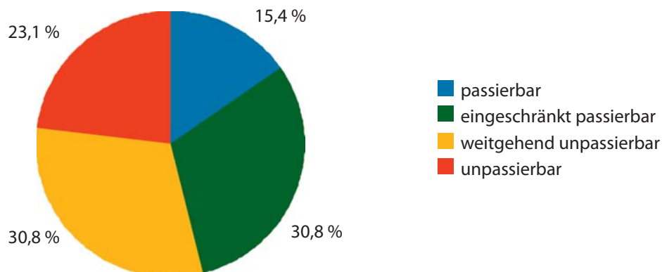
Abb. 77: Passierbarkeit der Querbauwerke für abwärts wandernde Fische im Höribach.
