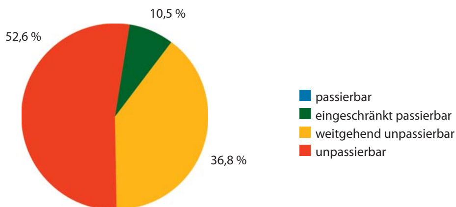
Abb. 43: Passierbarkeit der Querbauwerke für aufwandernde Fische in der Zeller Ache.
