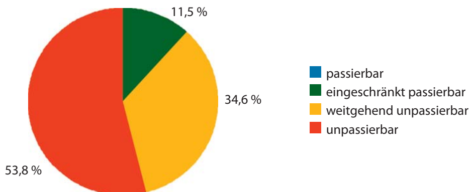
Abb. 32: Passierbarkeit der Querbauwerke für abwärtswandernde Fische im Pangraben.
