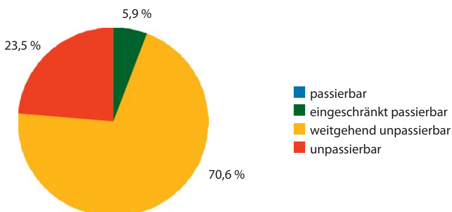
Abb. 53: Passierbarkeit der Querbauwerke für abwärtswandernde Fische im Kandlbach.
