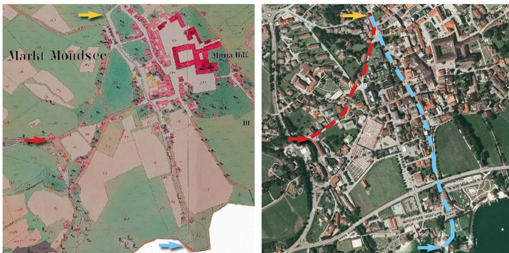
Abb. 130: Frühere oberflächliche (blaue Linie) und aktuelle unterirdische Führung (rote Linie) des Steinerbaches im Mondseer Ortsgebiet (links Franziszeischer Kataster (Franziszeische Landesaufnahme von 1824, © Land Oberösterreich, Original: Oö Landesarchiv), rechts Google Maps). Oranger Pfeil: Beginn der Verrohrung; roter Pfeil: heutige Mündung in die Zeller Ache; blauer Pfeil: frühere Mündung in den Mondsee.
