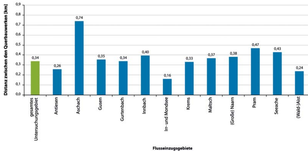
Abb. 10: Vergleich der durchschnittlichen freien Fließstrecken zwischen je zwei Querbauwerken in allen bislang untersuchten Flussgebieten.
