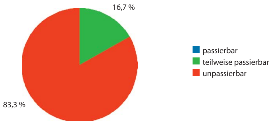
Abb. 38: Passierbarkeit der Querbauwerke für Benthosorganismen im Zeller Bach.
