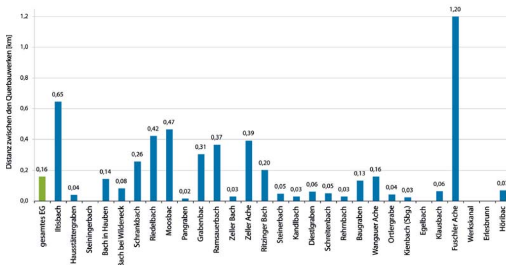
Abb. 9: Durchschnittliche freie Fließstrecke zwischen je zwei Querbauwerken [km] (EG = Einzugsgebiet).
