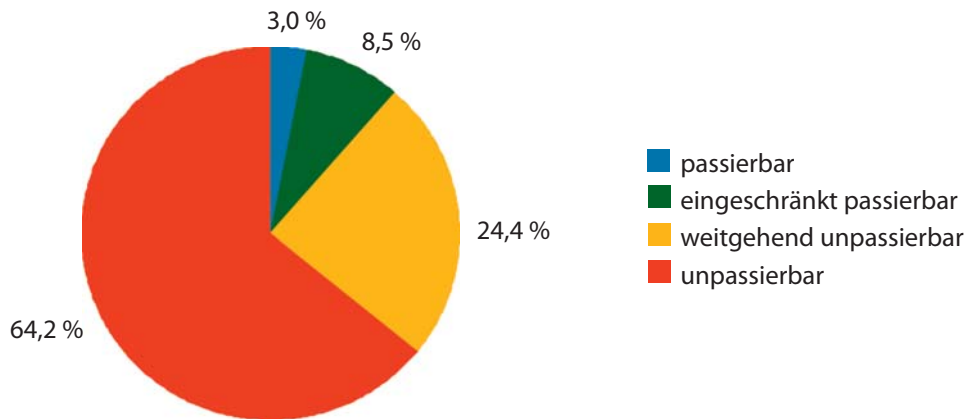
Abb. 15: Passierbarkeit der Querbauwerke für aufwärts wandernde Fische im Irr- und Mondsee-System.
