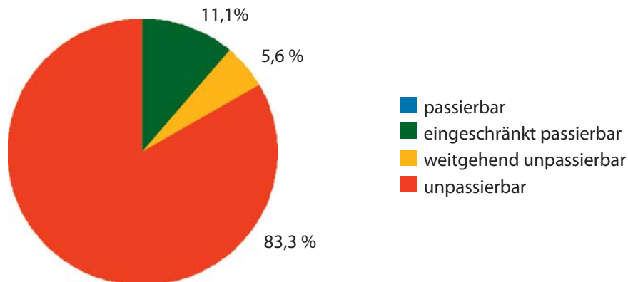
Abb. 36: Passierbarkeit der Querbauwerke für aufwandernde Fische im Zeller Bach.
