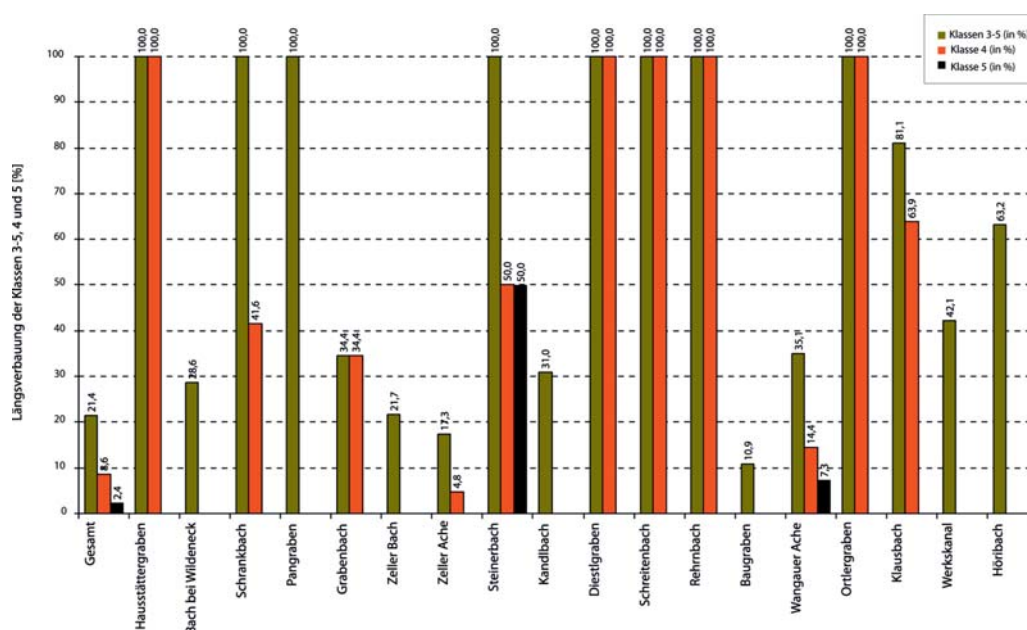
Abb. 81: Anteil der verbauten Uferlinie in Prozent der untersuchten Lauflänge pro Flusseinzugsgebiet der bisher erstellten Wehrkataster.
