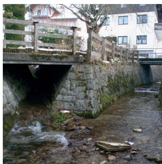
Abb. 123: Der Zeller Bach (rechts) ist im Ortsgebiet von Zell am Moos stark verbaut.
