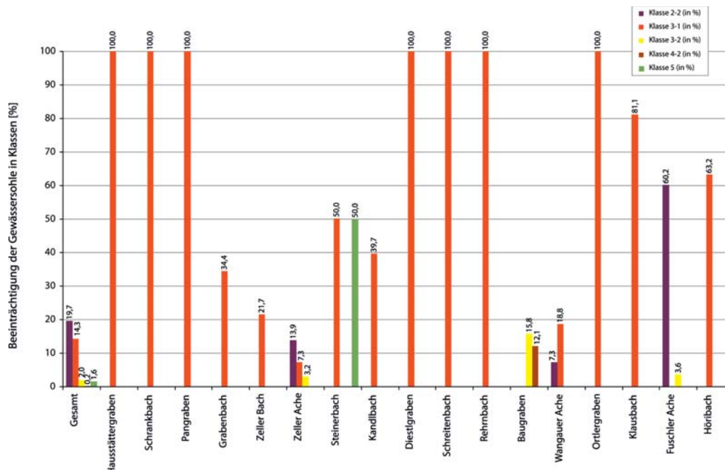
Abb. 80: Anteil der verbauten oder beeinträchtigten Gewässersohle in Prozent der untersuchten Lauflänge (Gesamt = gesamtes Einzugsgebiet).
