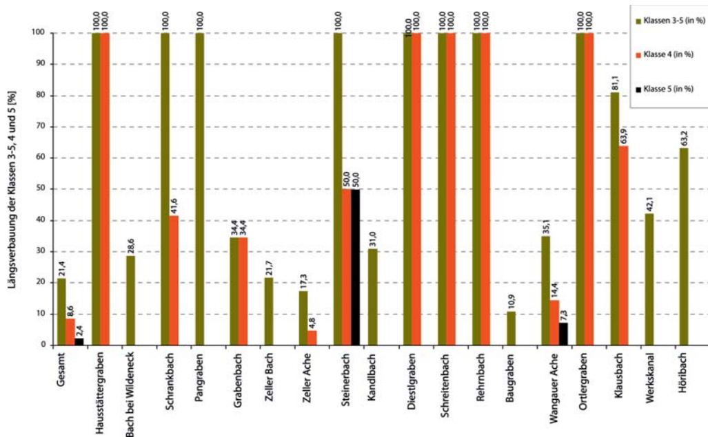
Abb. 79: Anteil der verbauten Uferlinie in Prozent der untersuchten Lauflänge (Gesamt = gesamtes Einzugsgebiet).
