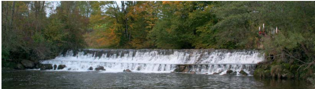
Abb. 7: Dieser Querbauwerksstandort verfügt über eine ganze Reihe konstruktiver Merkmale (siehe Text), die die Passierbarkeit verhindern (Foto: Fuschler Ache).
