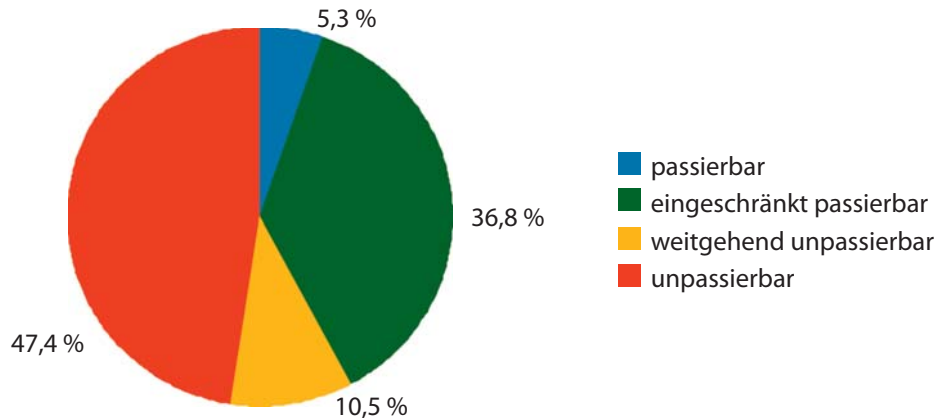
Abb. 44: Passierbarkeit der Querbauwerke für abwärtswandernde Fische in der Zeller Ache.
