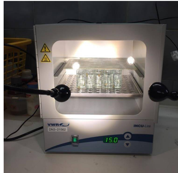
Abb. 5: Thermostat für Temperaturversuche
