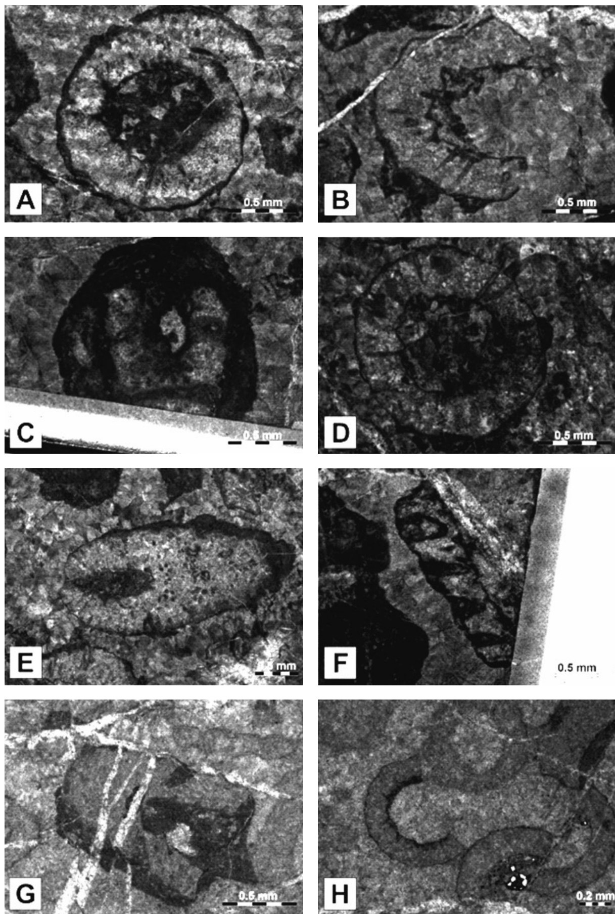
ABB. 11: Dasycladaceen aus dem Sengsengebirge (Probe 18/69/01: Schneetal) und von der Kremsmauer (Probe 17/68/20: Nordseite):
