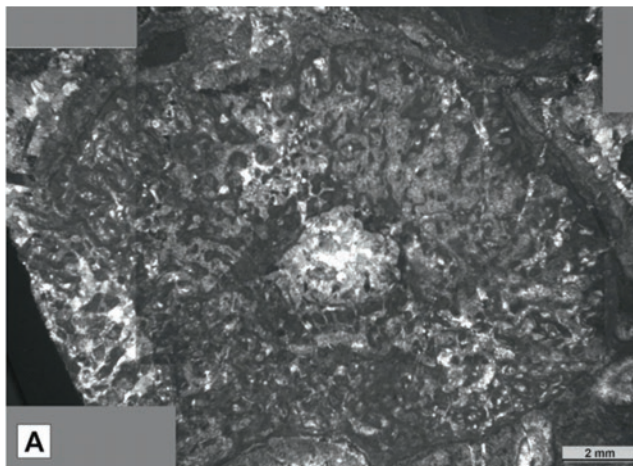
ABB. 19: Kalkschwämme von der Reilerschneid (1284 m): A: Dictyocoelia manon manon MÜNSTER; B: Vesicocaulis alpinus OTT
