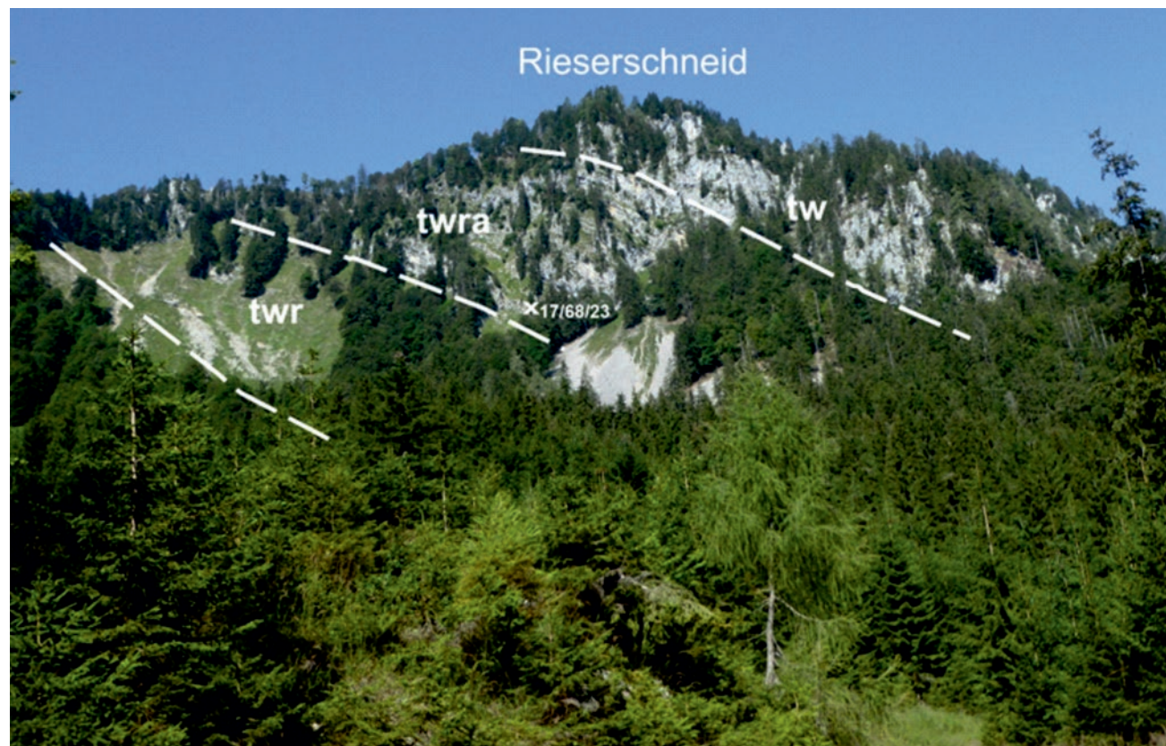
ABB. 18: Mitteltrias-Schichtfolge der Rieserschneid (1390 m): twr = Reifling-Formation, twra = Raming-Formation, tw = Wetterstein-Riffkalk; Lage der Probe 17/68/23 FIG. 18: Middle Triassic succession on mount Rieserschneid (1390 m); twr = Reifling Formation, twra = Raming Formation, tw = Wetterstein reef-limestone
