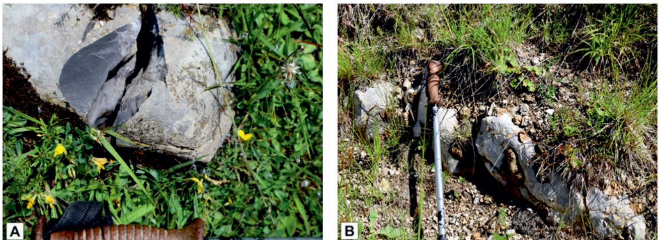
ABB. 23: Reifling-Formation am Großen Maierack (1764 m):
