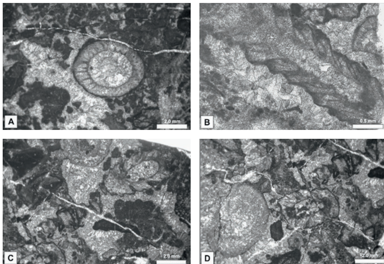
ABB. 4: Dasycladaceen vom Almkogel (A) und der Ackerschneid (B-D):
