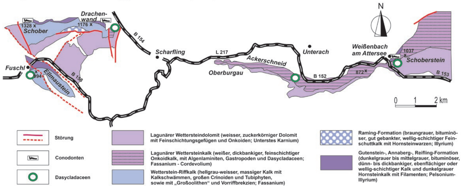
ABB. 3: Geologie der Mitteltrias zwischen Fuschlsee und Attersee
