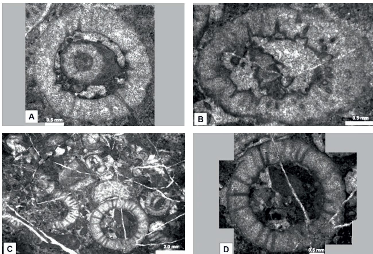
ABB. 6: Dasycladaceen aus dem Höllengebirge (380m SE' K. 1668, 1550m SH): A–D: Diplopora annulata annulata SCHAFFHÄUTL
