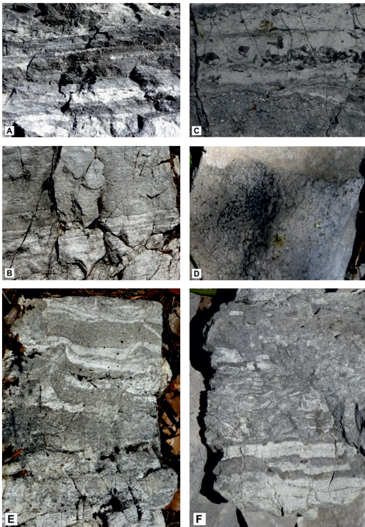
ABB. 13: Lagunärer Wettersteinkalk im Sengengebirge an der Südseite des Brettstein (1437 m):
