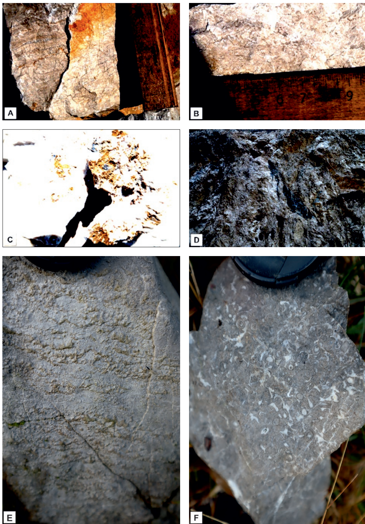
ABB. 14: Lagunärer Wettersteinkalk im Voest-Alpine Steinbruch Steyrling und lagunärer Wettersteinkalk am Schrattenstein bei Gmunden:
