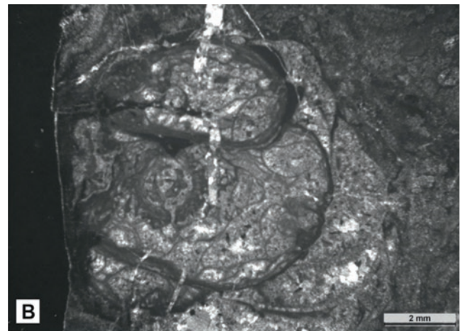
ABB. 19: Kalkschwämme von der Reilerschneid (1284 m): A: Dictyocoelia manon manon MÜNSTER; B: Vesicocaulis alpinus OTT
