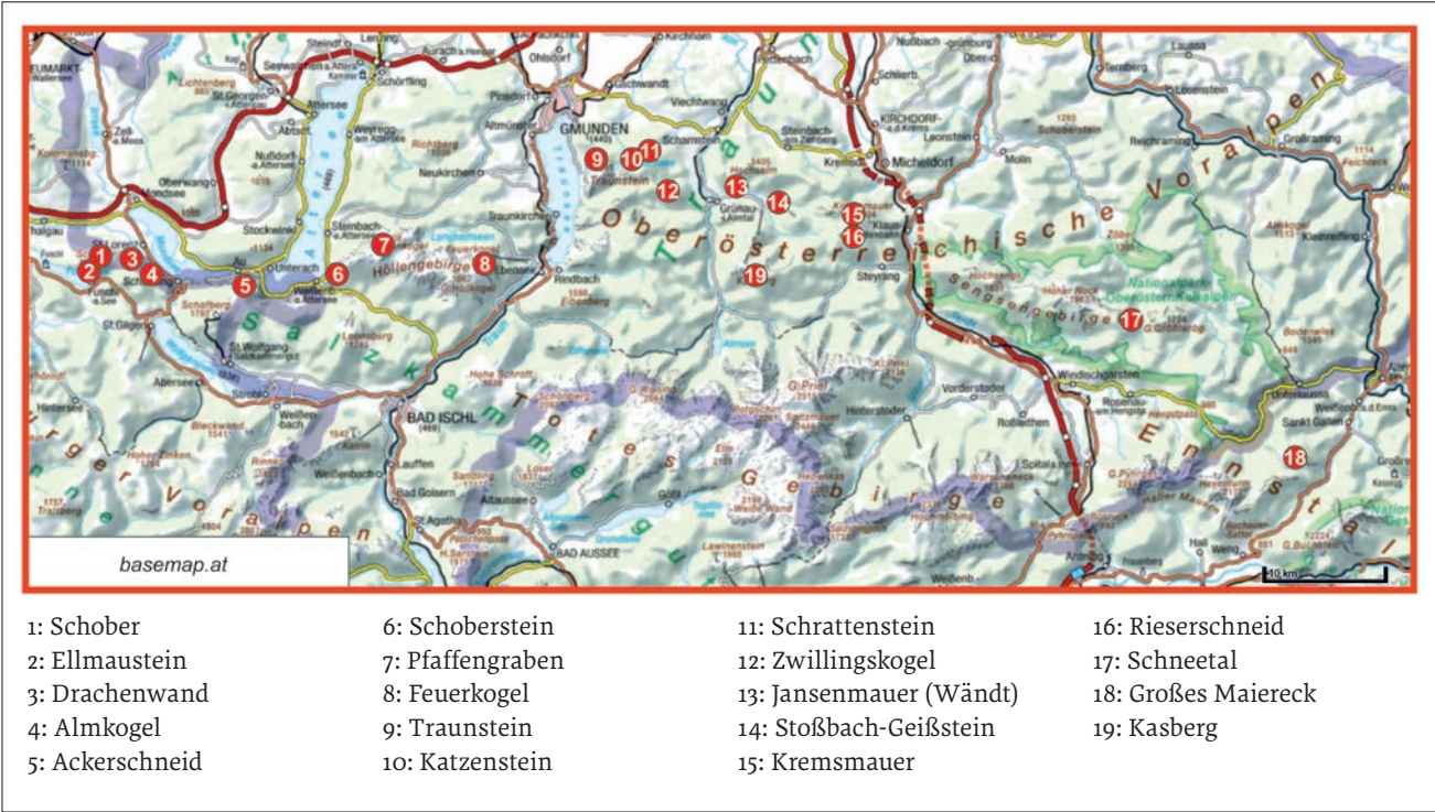
ABB. 1: Geografische Lage und Übersicht der Mitteltrias-Profil in Oberösterreich FIG. 1: Geographic overview and position of the different Middle Triassic sections in Upper Austria
