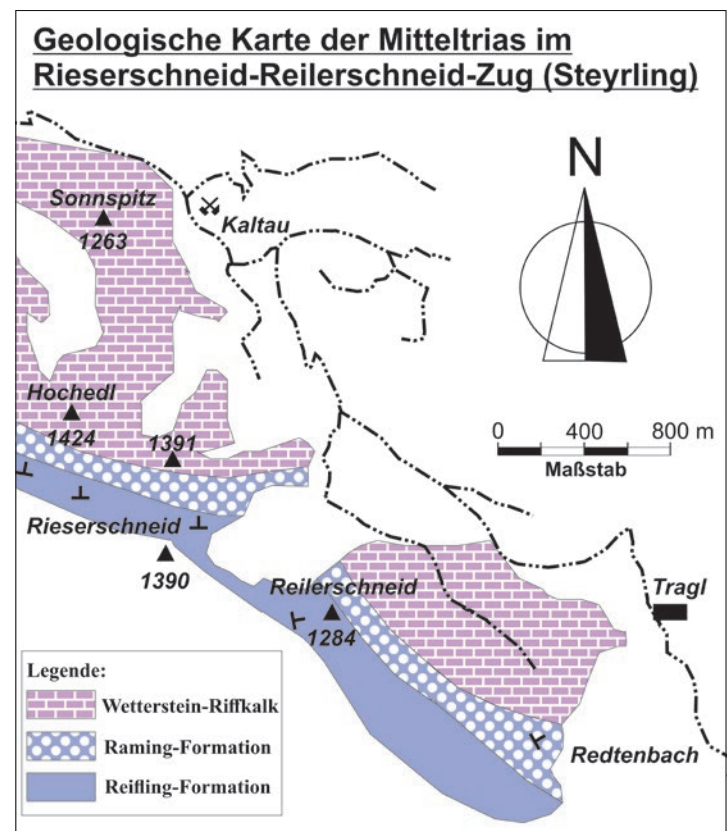
ABB. 20: Geologische Karte Kaltau FIG. 20: Geological Map Kaltau
