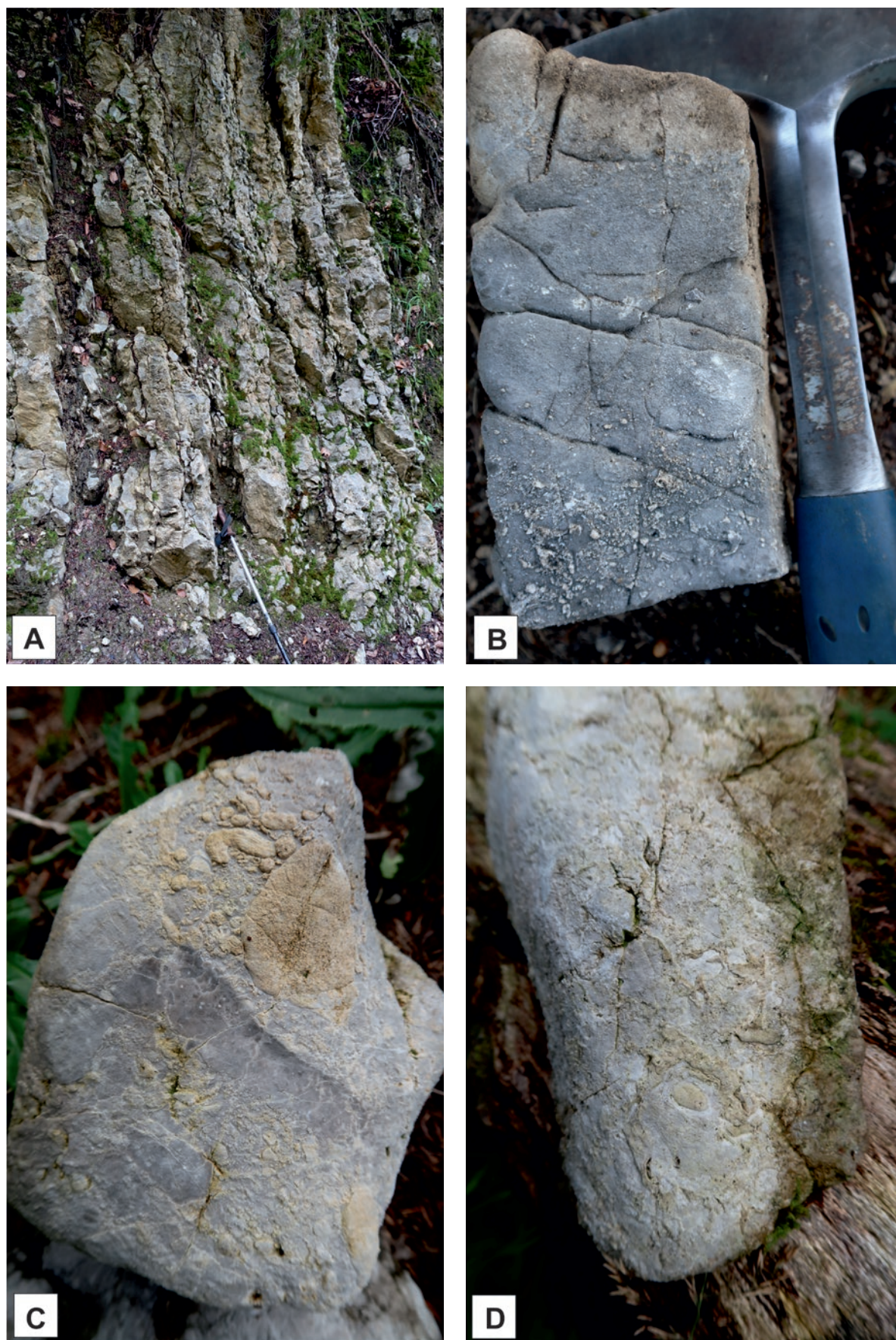
ABB. 16: Stoßbach und Zwillingskogel (1402 m):
