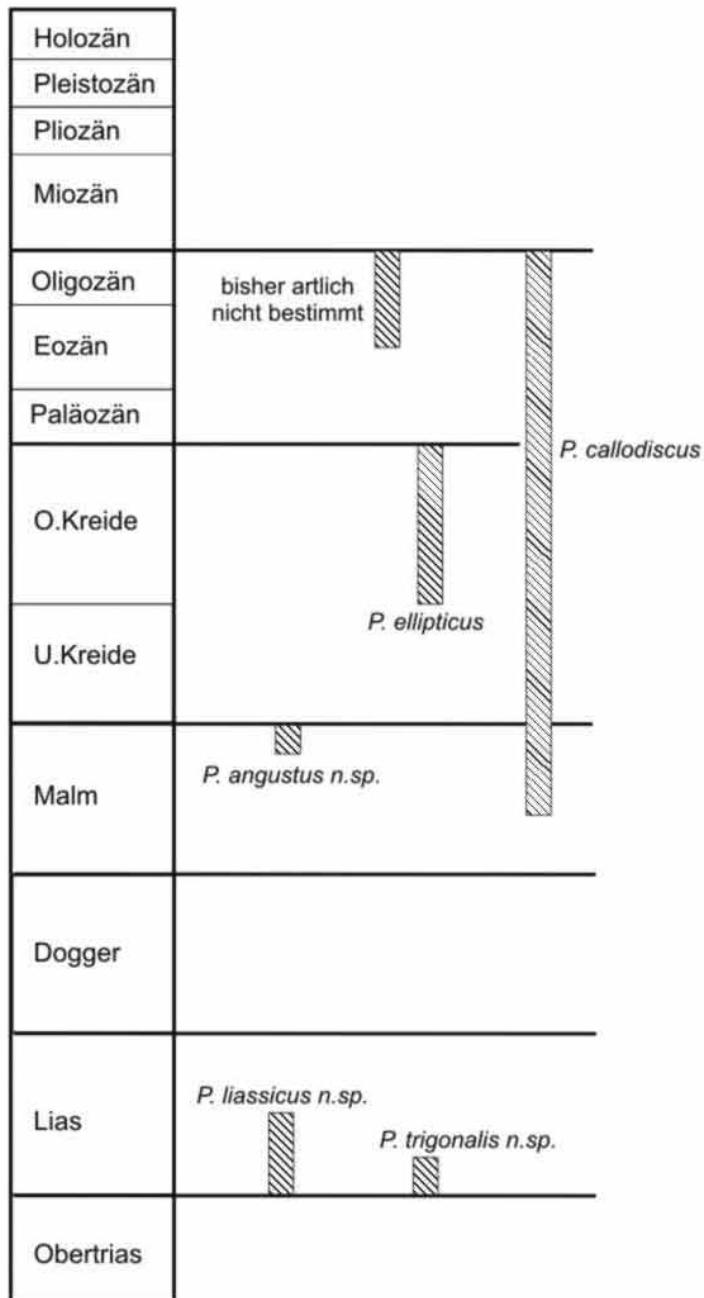
Abbildung 5: Stratigraphische Verbreitung der Prodactylolalicytes Arten
