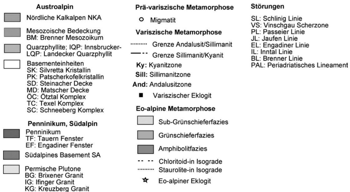
Abb. 2: Schematische Metamorphosekarte des westlichen Austroalpins; schwarz eingrahmt ist die Begrenzung des Bergbaureviere Pflersch-Schneeberg. Das weiße Rechteck stellt das bearbeitet Gebiet im Lazzachertal dar. SNFZ: Schneeberg normal fault zone.
