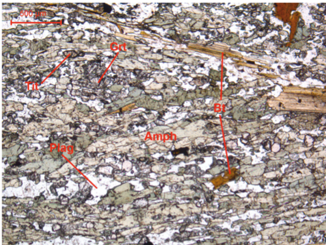
Abb. 6: Granatführender Amphibolit aus dem Lazzachertal bei //N. Die grünlichen Hornblendens (Amph) stellen den größten Anteil an der Mineralparagenese dar. Untergeordnet treten Granat (Grt), Plagioklas (Plag), Biotit (Bt) und Titanit (Tit) auf.
