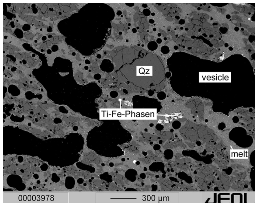
Abb. 7: Probe VT8. Das BSE Bild zeigt das typische Gefüge eines pyrometamorph überprägten Diorits (Klausenit) mit einer auffallend großen Porosität des Gesteins. Zudem sind im Quarz (Qz), eine große Menge an Schmelze (melt) und die Ti-Fe-Phasen, bestehend aus Ilmenit, Magnetit, Rutil und Herzynit, erkennbar. Grosse Löcher (vesicle) sind ebenfalls erkennbar.
