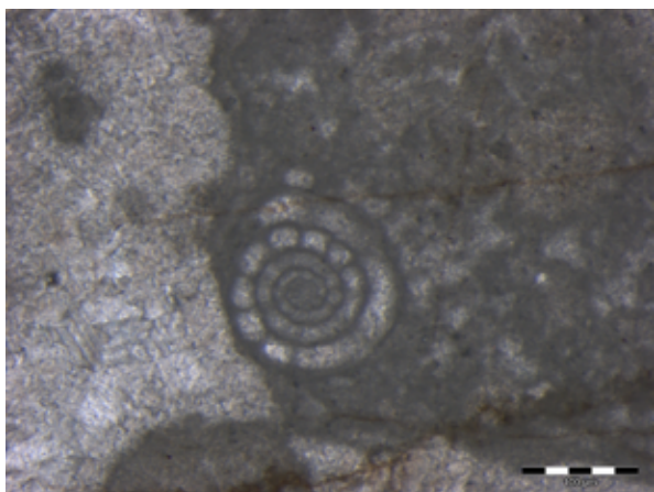
Abb. 7: Meandrosira dinarica Kochansky-Devide & Pantić; Lokalität: Jagdsteig 490 m W' K. 841 Balkenlänge: 0.1 mm
