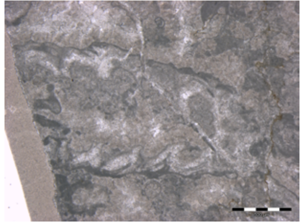
Abb. 4: Physoporella pauciforata gomerica Bystrický; Lokalität: Wanderweg 190 m SE' K. 841 Balkenlänge: 0.5 mm
