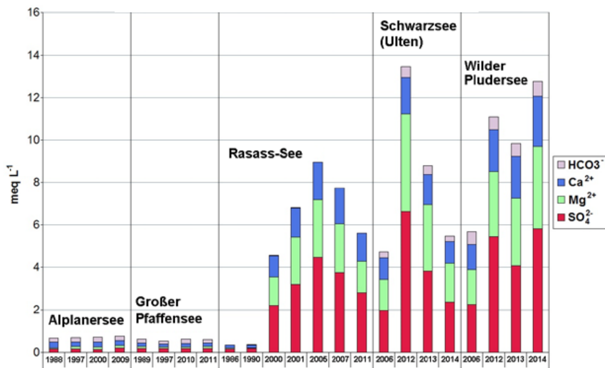
Abb. 6: Langzeitentwicklung der Hauptionenzusammensetzung in blockgletscherbeeinflussten (Rasass-See, Schwarzsee und Wilder Pludersee) und in unbeeinflussten Seen (Alpanersee und Großer Pfaffensee).
