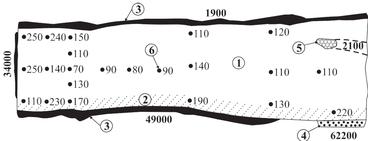
Abb. 37. Schnitt durch einen plattigen Klufkörper des Labiatus-Pläners (Größe ca. 60 \times 7 cm, senkrecht zur Schichtung). 1: Kalkstein bis Mergelstein, dunkelgrau, äußerlich unverändert; 2: Kalkstein bis Mergelstein, leicht braun verfärbt; 3: Kluftbelag, dunkelbraun bis schwarzbraun, gelartig erstarrt; 4: Kluftbelag, weiß, gelartig erstarrt; 5: röhrenförmiger Hohlraum, gefüllt mit dunkelbraunen bis gelbbraunen Eisenoxiden/-hydroxiden; 6: Probe, Aktivitätskonzentration für U-238 [Bq/kg].
