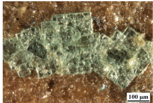
Abb. 30. Zeunerit-, Metazeunerit (Lagerstätte Culmischer, Zechstein).
