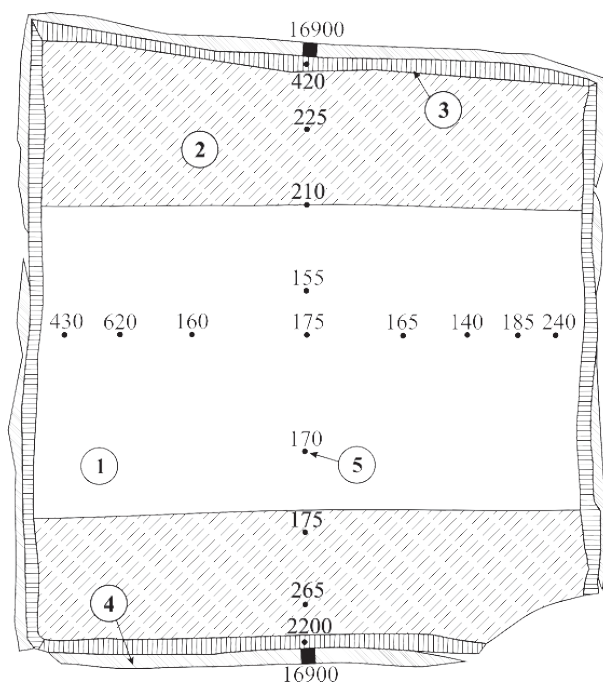
Abb. 38. Schnitt durch einen Klufkörper des Labiatus-Pläners (Größe ca. 5 \times 5 cm, senkrecht zur Schichtung). 1, Kalkstein bis Mergelstein, grau, äußerlich unverändert; 2, Kalkstein bis Mergelstein, hellgraubraun verfärbt; 3, Reaktionssaum des Gesteins an den Klufflächen, braun bis dunkelbraun; 4, Kluftbelag, dunkelbraun bis schwarzbraun, partiell gelbbraun, gelartig erstarrt; 5, Probe, Aktivitätskonzentration für U-238 [Bq/kg].
