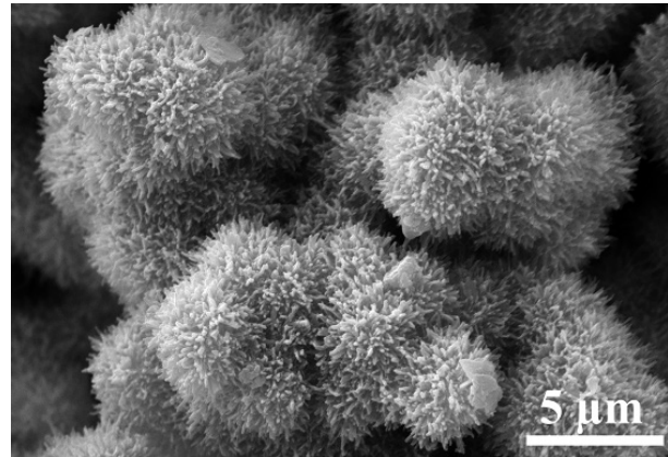
Abb. 11. Igelartige Sphäroide von Natriumboltwoodit.
