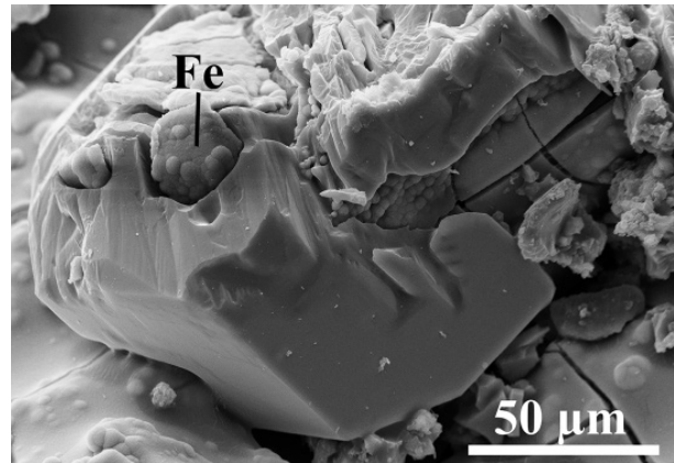
Abb. 40. Uranhaltiger Eisenhydroxid-/oxideinschluss (Fe) in einem Gipskristall (Tab. 1, Spalte 31).
