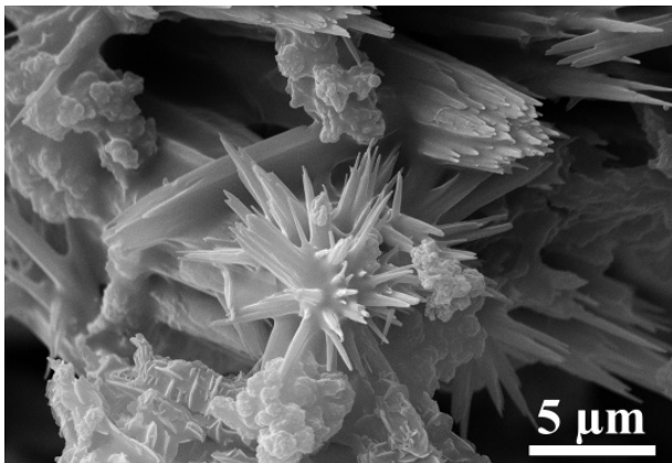
Abb. 25. Calciumkarbonatnadeln (Zentrum) mit Sklodowskitaggregaten (oberhalb und unterhalb).
