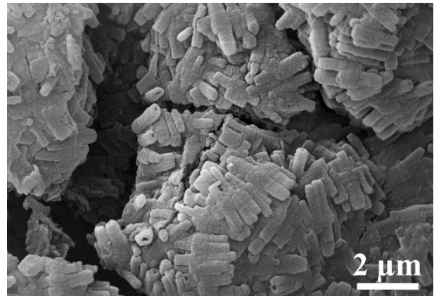
Abb. 23. Sekundäre Kieselsäurekruste – Aggregat röhrenförmiger Kristalle.
