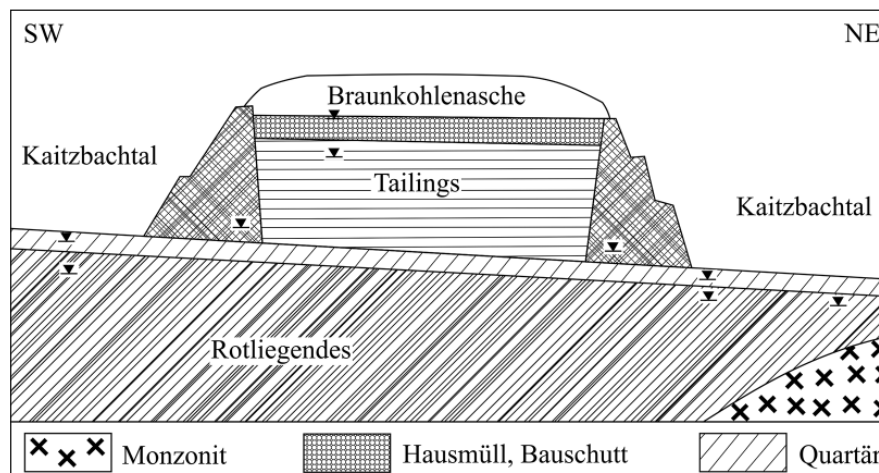
Abb. 2. Schematischer Schnitt durch die Halde A. Fig. 2. Schematic cross-section through the tailings dump A.
