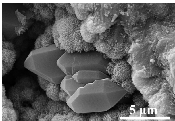
Abb. 28. Goethitaggregat mit idiomorphen Quarzkristallen im Hohlraum einer verwitterten Pyritkoncretion.
