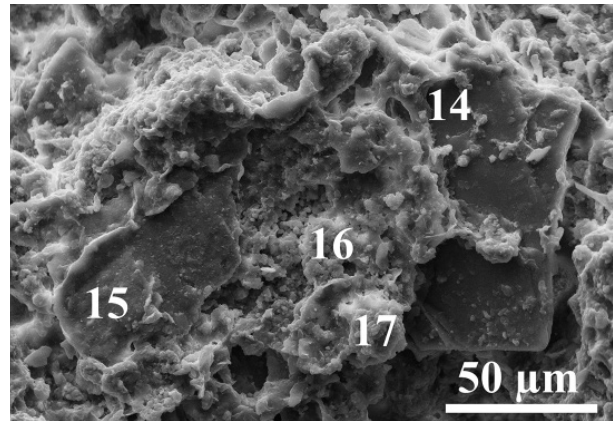
Abb. 19. Alteration eines Glimmerpaketes durch Säure (Spalten 14 bis 17 in Tab. 1).
