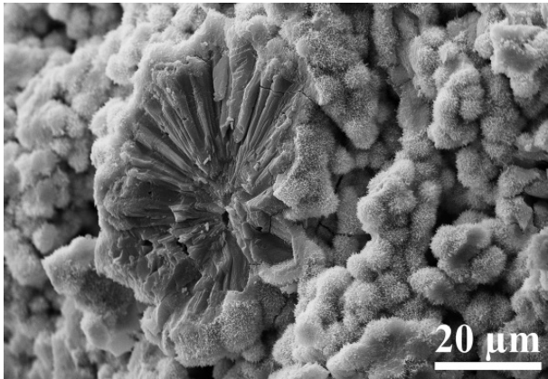
Abb. 10. Natriumboltwooditkruste auf einem Calciumcarbonataggregat.
