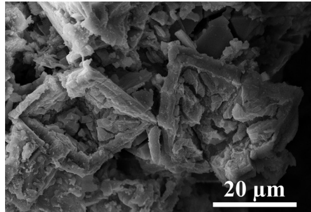
Abb. 47. In Goethit umgewandelter Pyrit in einer alterierten Pyritkoncretion im Turon-Pläner.
