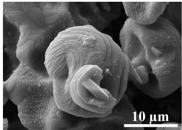
Abb. 17. Jarositektallbildung auf der Oberfläche des Jarositgels.
