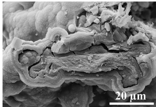
Abb. 42. Beispiel für den lagenförmigen Aufbau einer gelartigen Kruste auf einer Kluftfläche im Turon-Pläner.
