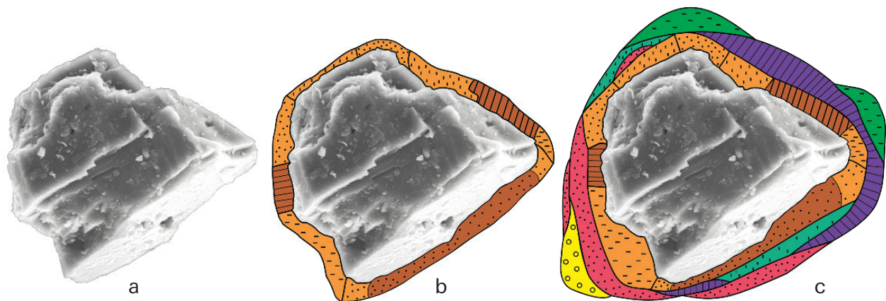
Abb. 50. Schematische Darstellung der Bildungsphasen eines Adsorptionsmischkristalles in den Tailings der Halde A. a: Feldspatkern; b: Fällung und Anlagerung der ersten Schicht an den Kern; c: Anlagerung weiterer Schichten.
