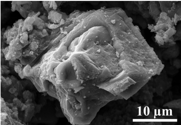
Abb. 46. Korrodierter Pyritkristall in einer Pyritkoncretion im Turon-Pläner.
