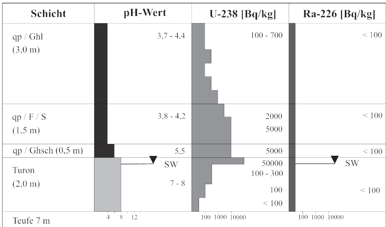
Abb. 33. Fällung von U-238 an der Grenze Quartär Kreide durch Neutralisation (Halde A; qp, Quartärsedimente; SW, Sickerwasser).
