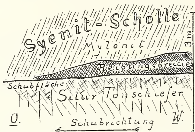
Figur 5. Der Überschiebungskontakt auf der Südseite des Kukkesvagge unterhalb des Buchtsgletschers.
