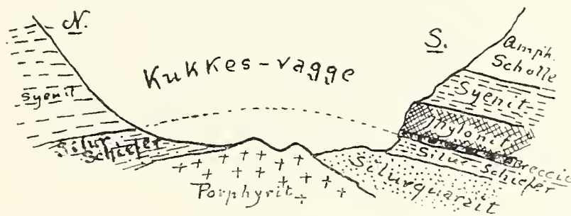
Figur 4. Profilskizze der Lagerungsverhältnisse im Fenster der Kukkesvágge (Die Überschiebungsfäche ist durch die punktierte Linie angedeutet.)
