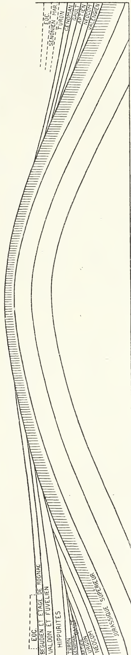
Schematischer Querschnitt durch die Basse-Provence, die relative Lage der Kreidesedimente und damit die Randzonen des Kreidemeeres zeigend. (Abgeändert aus Collot.)
