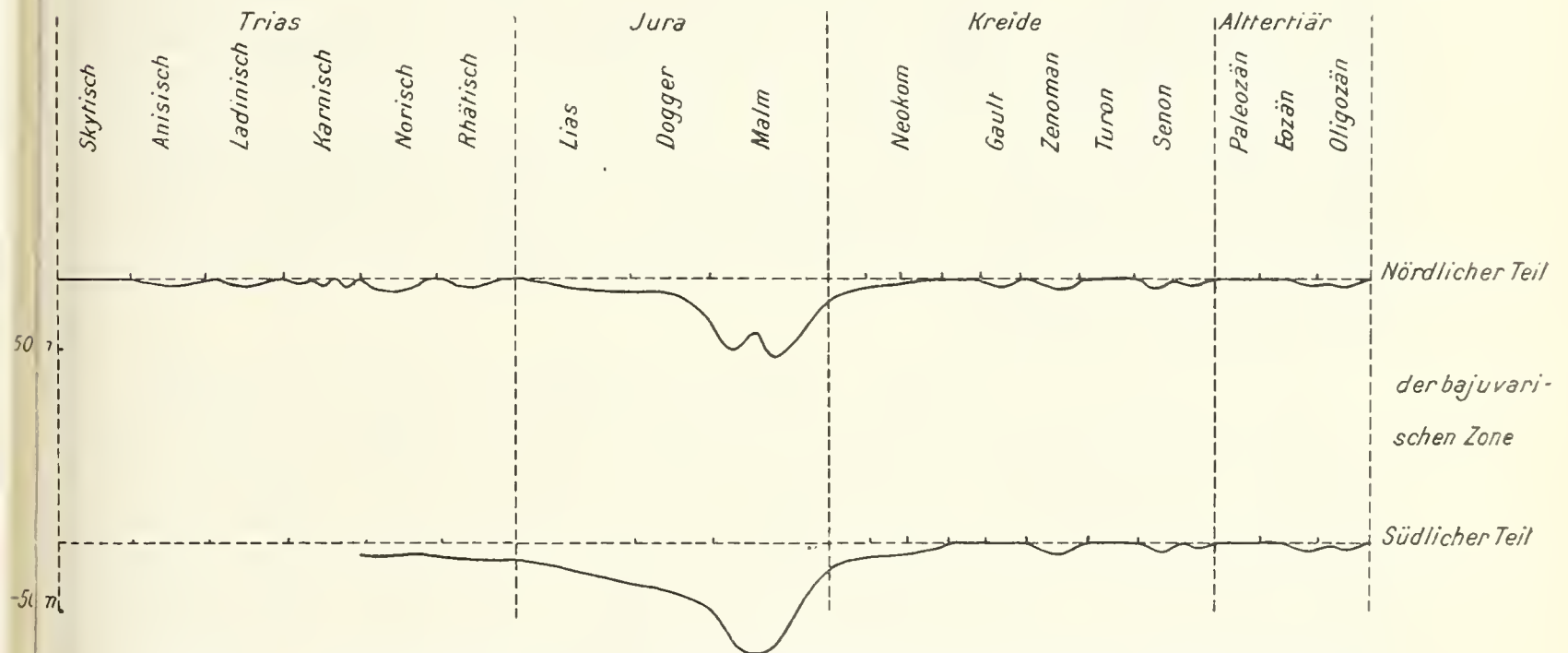
Fig. 1. Tiefendiagramm der Meeresbedeckung in der bajuvarischen Zone.
