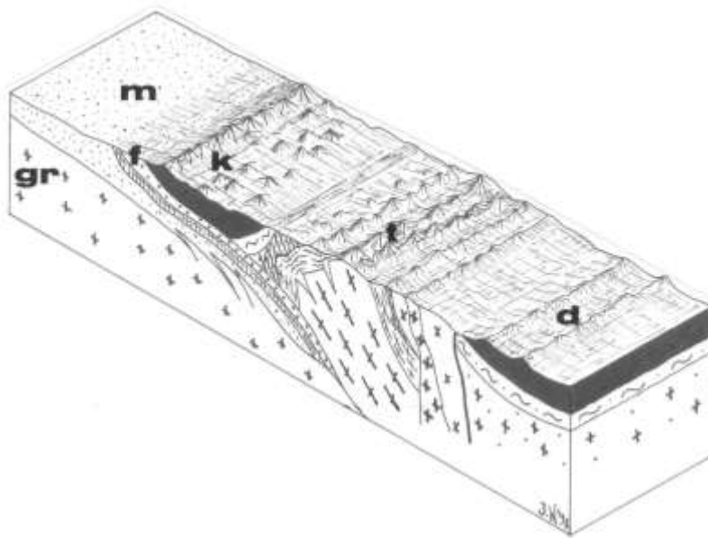
Abb. 7: Vereinfachter geologischer N-S Schnitt durch die Alpen heute; Granite der Böhmisches Masse (gr); Kalkalpen (k) samt Gosauschichten liegen über (gr), Molasse (m) und Flysch (f); nach Süden schließen die Hohen Tauern (t) und die Dolomiten (d) an.
