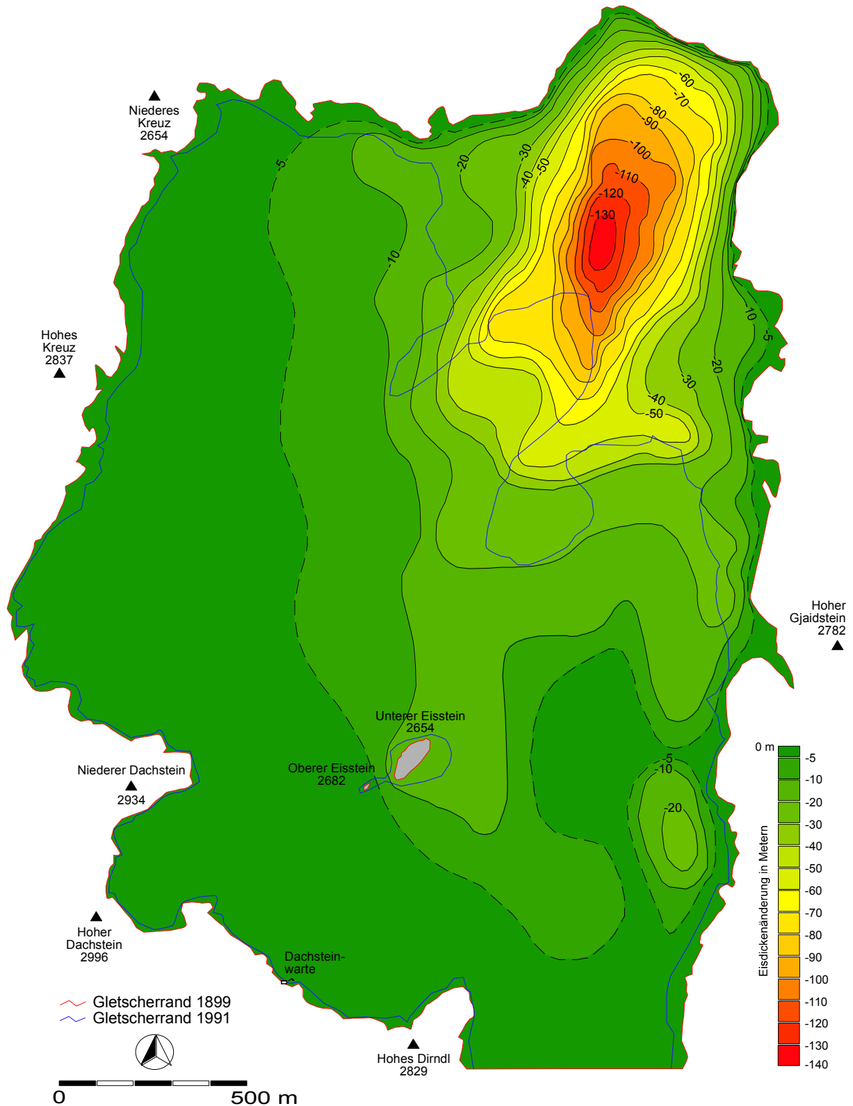
Abb. 6: Eisdickenänderung am Hallstätter Gletscher zwischen 1899 und 1991
