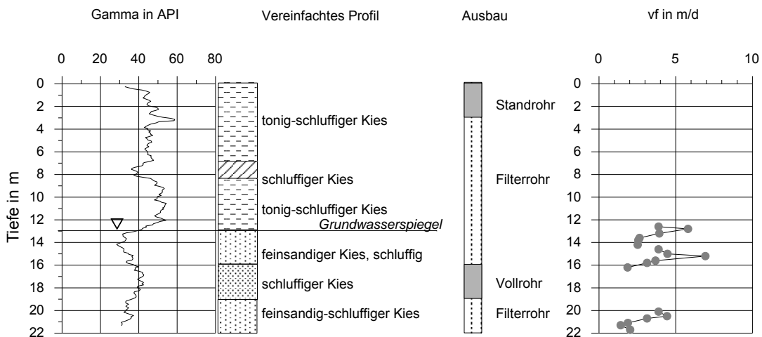
Abb. 3: Aufschlussbohrung „Heiliges Bründl“ mit Gammalog, vereinfachtem geologischen Profil, Ausbauschema und Ergebnissen der Messungen mit der Thermosonde
