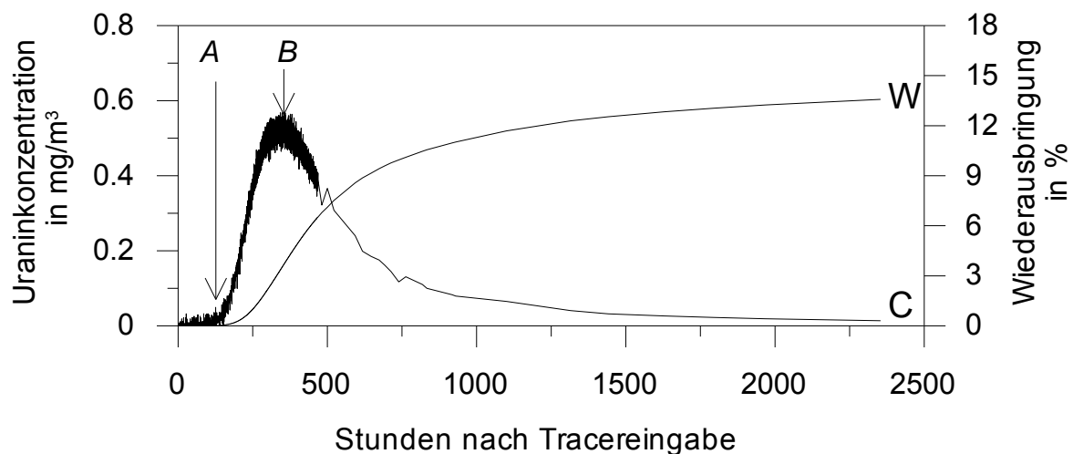
Abb. 5: Zeit-Konzentrationsdiagramm mit Uranin-Durchgangskurve (C) und Kurve des Wiederausbringens (W); A markiert das erste Auftreten (86,5 Stunden), B das Durchgangsmaximum (343 Stunden)
