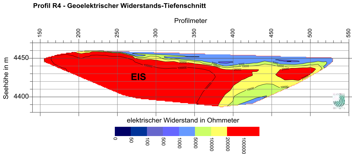
Abbildung 12: Widerstandstiefensektion der geoelektrischen Messungen am Profil R4 – ein ausgedehnter Permafrostbereich, erkennbar an den sehr hohen Widerständen von über 20 000 Ohmm tritt deutlich hervor. (Joanneum Research 1999)
