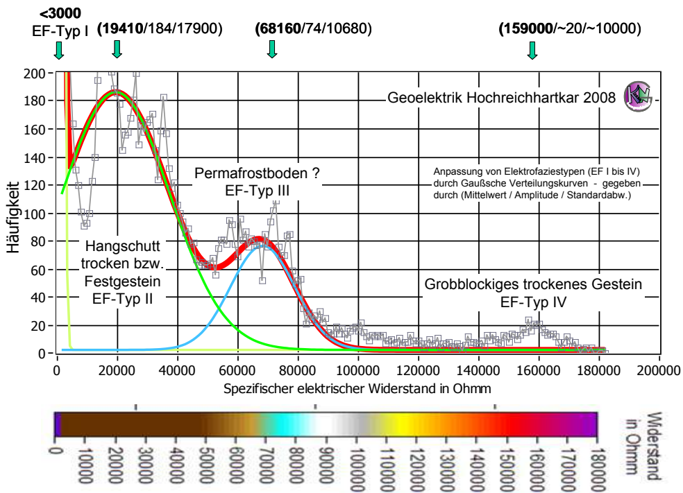
Abb. 4: Histogramm der elektrischen Widerstände am Messprofil und Zuordnung zu Elektrofaciestypen.
