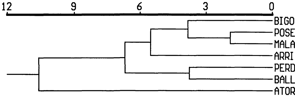
Fig. 5: UPGMA dendrogram based on Mahalanobis distances of grouped female Iberolacerta bonnali samples (see table 8). Abb. 5: UPGMA dendrogram auf Grundlage der Mahalanobisdistanzen zwischen den gruppierten Iberolacerta bonnali Weibchen-Stichproben (siehe Tab. 8).
