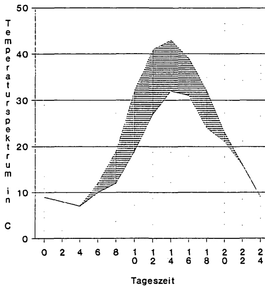
Abb. 4: Ouarzazate (Marokko). Schatten- und Sonnentemperaturen im Tageslauf des 12.04.1982 (nach Messungen des Verfassers).
