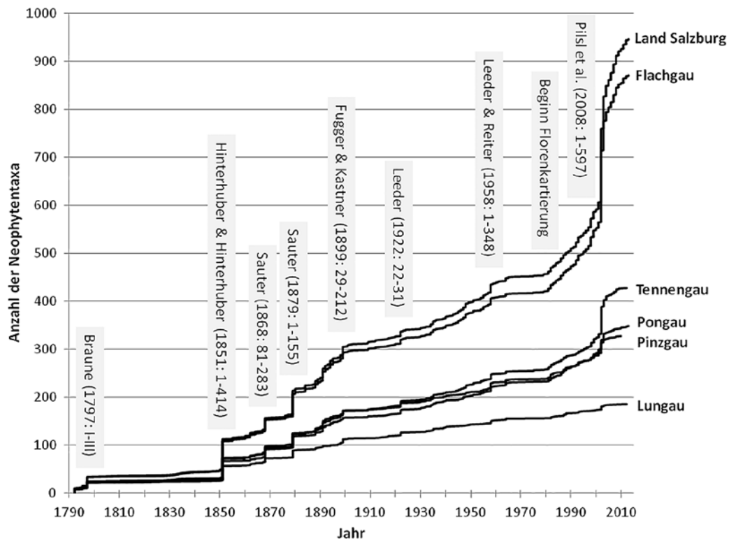
Abb. 2: Anzahl der dokumentierten Neophyten taxa von 1790 bis 2013. Diese sind für das gesamte Bundesland, als auch für die einzelnen Gaue in einem Liniendiagramm dargestellt. Zusätzlich werden wichtige floristische Ereignisse (grau hinterlegt) erwähnt, welche zu einem deutlichen Anstieg der Neophytenanzahl geführt haben.
