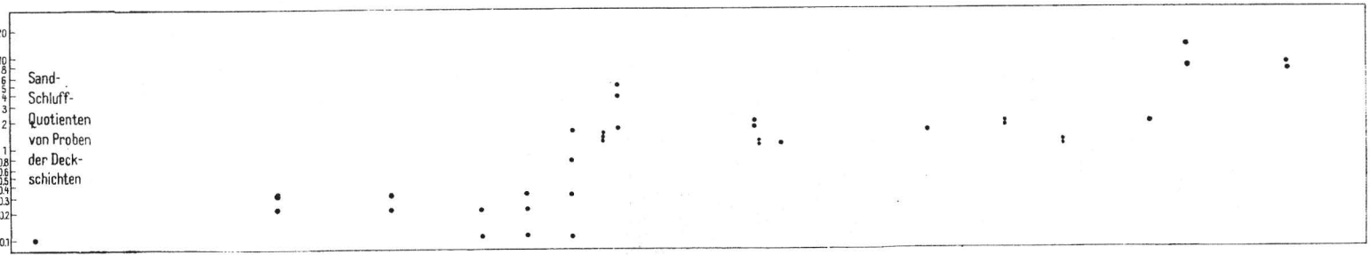
Abb. 11. Schematische Darstellung des Profilschnittes Zörbig (Lage s. Abb. 1) mit Korngrößenzusammensetzung (Blockdiagramme) der typischen Profile und Sand/Schluff-Quotienten der Deckschichten der untersuchten Profile
