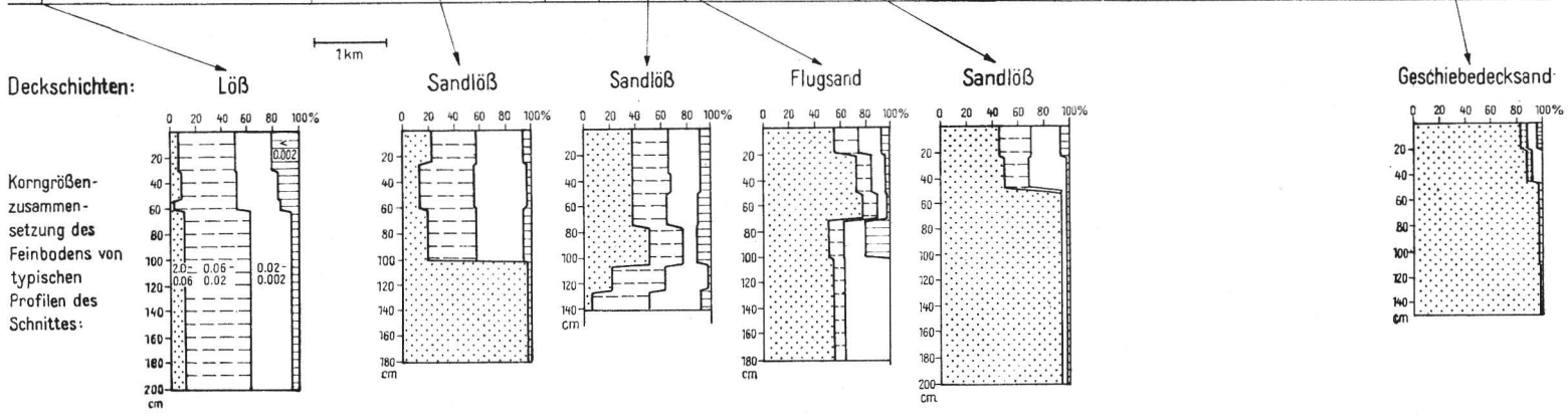
Abb. 11. Schematische Darstellung des Profilschnittes Zörbig (Lage s. Abb. 1) mit Korngrößenzusammensetzung (Blockdiagramme) der typischen Profile und Sand/Schluff-Quotienten der Deckschichten der untersuchten Profile
