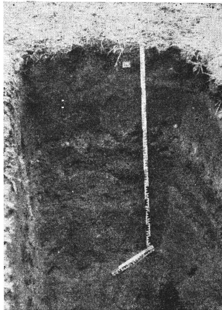
Abb. 8. Beispiel für eine geringmächtige Sandlößdecke mit Steinsohle an der Basis der Deckschicht
