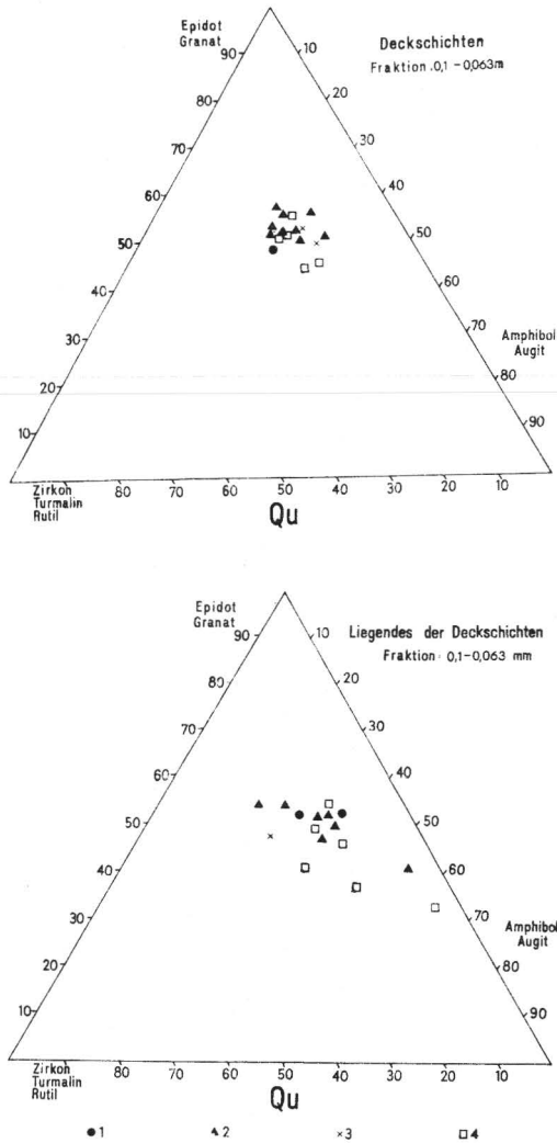
Abb. 14. Beispiele für Dreiecksdiagramme der Schwermineralverteilung der Deckschichten und der Liegendensedimente
