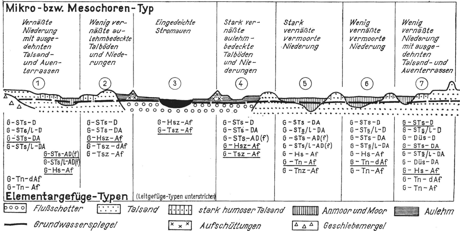
Abb. 2. Ausstattung und Abfolge von Naturraumtypen in den Tälern und Niederungen des Tieflandes der DDR (schematisches überhöhtes Profil)
