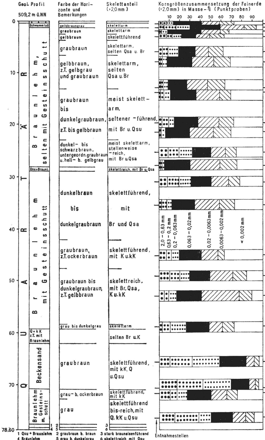
Abb. 11. Geologisches Profil, Korngrößenzusammensetzung und Chemismus der Kernbohr-
