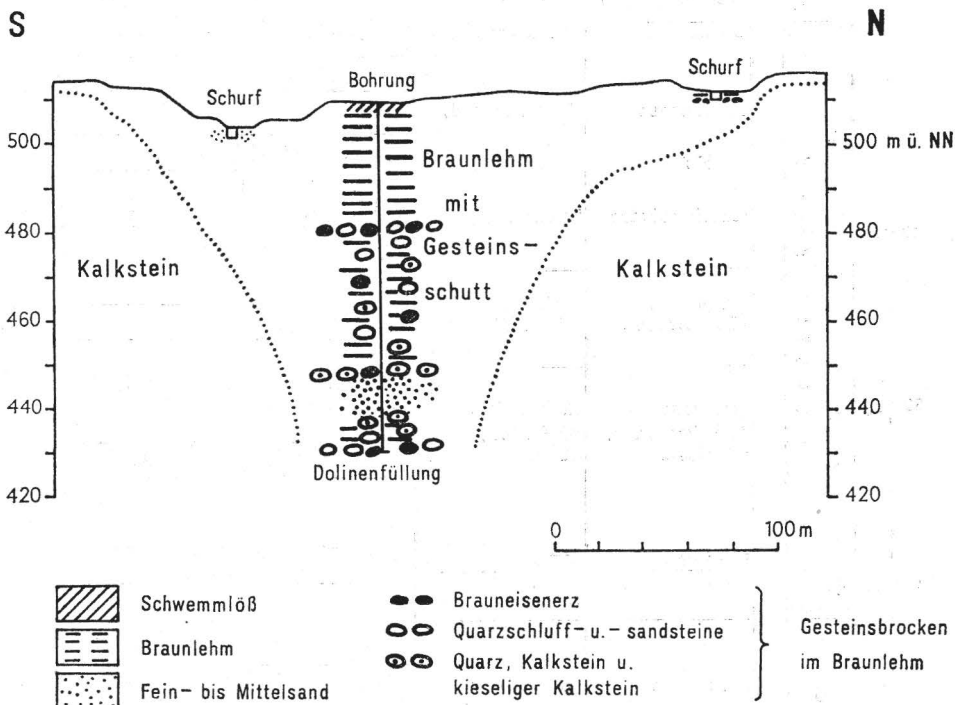
Abb. 10. Schematischer Schnitt durch die Doline am Kleinen Schmidtkopf (s. Abb. 1; detaillierte Darstellung der Bohrung s. Abb. 11)
