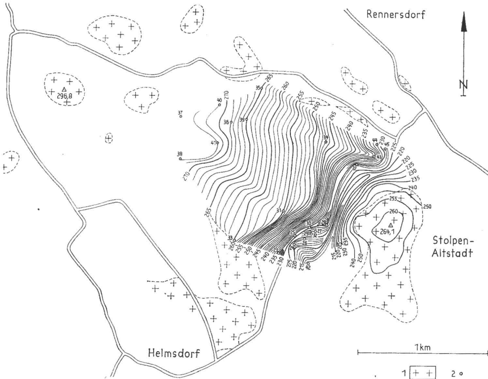
Abb. 6. Isohypsenskarte der Granodioritoberfläche 1 Granodioritausstriche, 2 Bohrungen
