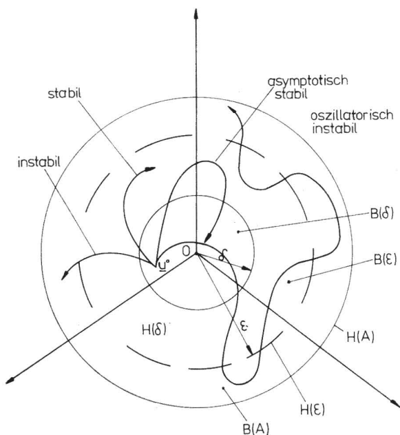
Abb. 5. Stabilitätsuntersuchung des Koordinatenursprungs. Die einzelnen möglichen Bewegungen des Systems beginnen stets im Koordinatenursprung ( u^* -Anfangszustand). 0-Koordinatenursprung, \delta , \varepsilon -Stabilitätsgrenzen, B(\varepsilon) -Bereich \|u\| < \varepsilon , H(\varepsilon) -Hülle des Bereiches \|u\| = \varepsilon , B(\delta) -Bereich \|u\| < \delta , H(\delta) -Hülle des Bereiches \|u\| = \delta , B(A) -Bereich \|u\| < A , H(A) -Hülle des Bereiches \|u\| = A
