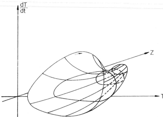
Abb. 13. Beurteilung der Systembewegung anhand des Trajektorienverlaufes der Größe Wassertemperatur im Pelagial der Talsperre Saidenbach. Mit zunehmender Tiefe z werden die Amplituden der Temperaturgradienten kleiner. Weitere Erläuterungen im Text
