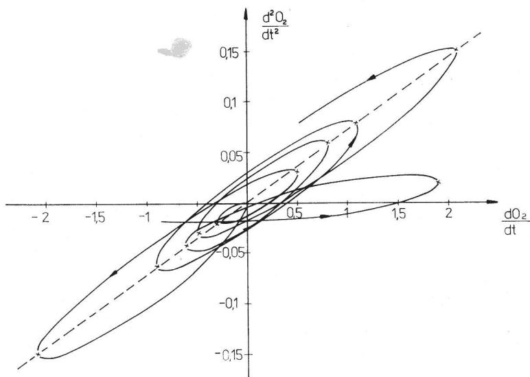
Abb. 11. Sensitivität der Größe Sauerstoffgehalt. Die Amplitude des Gradienten ändert sich im saisonalen Rhythmus. Die Änderung erfolgt in der durch die unterbrochene Gerade angedeutete Ebene (Obere Talsperre Neunzehnhain, Entnahmetiefe der Wasserproben 5 m, Durchschnittskurve der Jahre 1966–1970)
