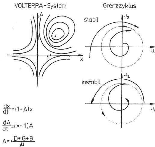
Abb. 6. Gleichgewichtsschnittpunkt eines Ökosystems außerhalb des Koordinatenursprungs (Volterrasystem) als Beispiel des Trajektorienverlaufes bei nichtlinearen Systemen. Schematische Darstellung eines stabilen und eines instabilen Grenzzyklus
