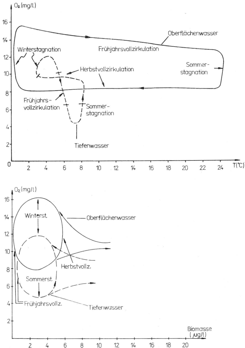
Abb. 8. Zustandsdiagramme von Teilsystemen eines Talsperrenökosystems. a) Teilsystem Wassertemperatur/Sauerstoffgehalt, b) Teilsystem Phytoplanktonbiomasse/Sauerstoffgehalt, jeweils für den Oberflächenwasser- und Tiefenwasserbereich des Pelagials der Talsperre Saldenbach
