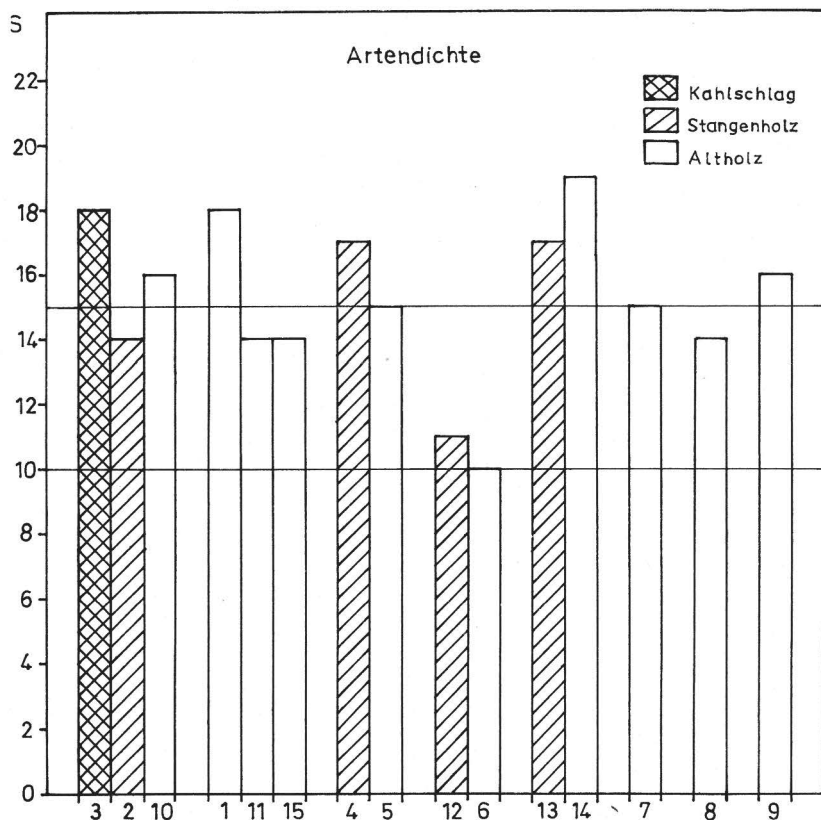
Abb. 2. Die Artendichten der untersuchten Carabidenzönosen des Hakel
