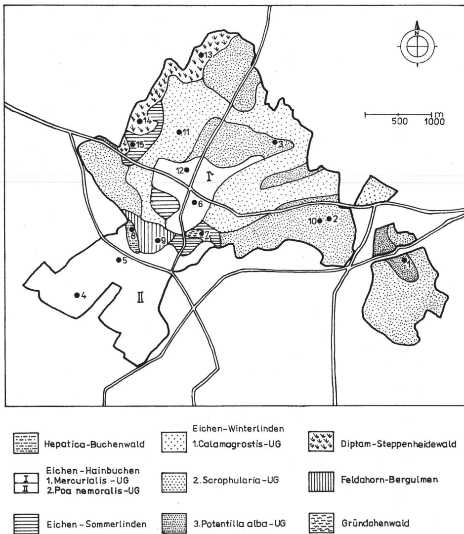
Abb. 1. Die Waldgesellschaften des Havel nach Weinitschke (1954) sowie die Standorte (Nr. 1 bis 15) der Barberfallen 1879.
