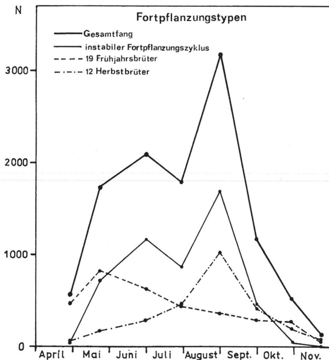
Abb. 8. Jahresrhythmik der Gesamtaktivität der verschiedenen Fortpflanzungstypen der Carabiden im Hakei
