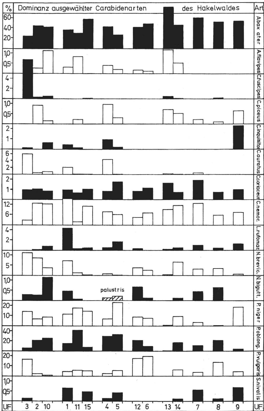
Abb. 4. Dominanz ausgewählter Carabidenarten auf den verschiedenen Waldstandorten im Hakei
