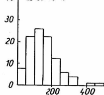
Abb. 1 Granit I II III IV 23 20 46 11
