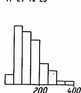
Abb. 2 Granit I II III IV 11 27 42 23
