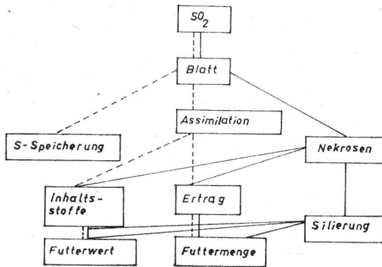
Abb. 1. Wirkungskette \text{SO}_2 nach (Däpfler 1971)
