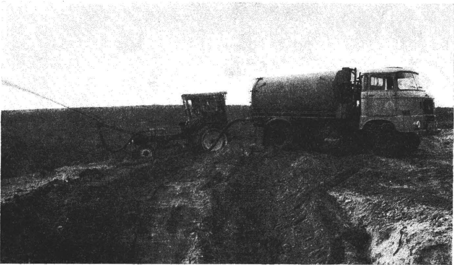
Abb. 6. Anspritztechnik im Einsatz (Foto: Dr. Schoppe)
