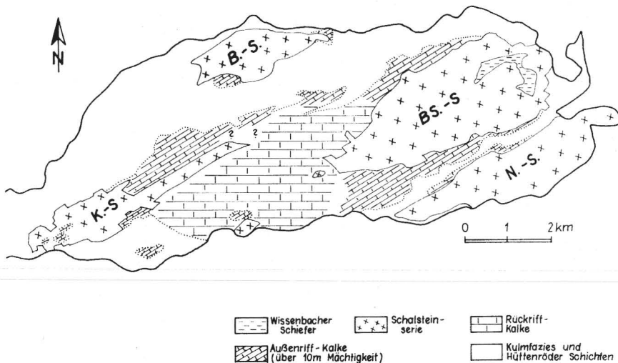
Abb. 2. Generalisierte Karte des Elbingeröder Komplexes mit den Vulkanitaufbrüchen von Neuwerk (N-S.), Braunesumpf (BS-S.), Büchenberg (B-S.) und Königshütte (K-S.) und mit der Verbreitung der Rückriff- (Atollstadium) sowie der Außenriffkalke (Atoll- und Kappenstadium)
