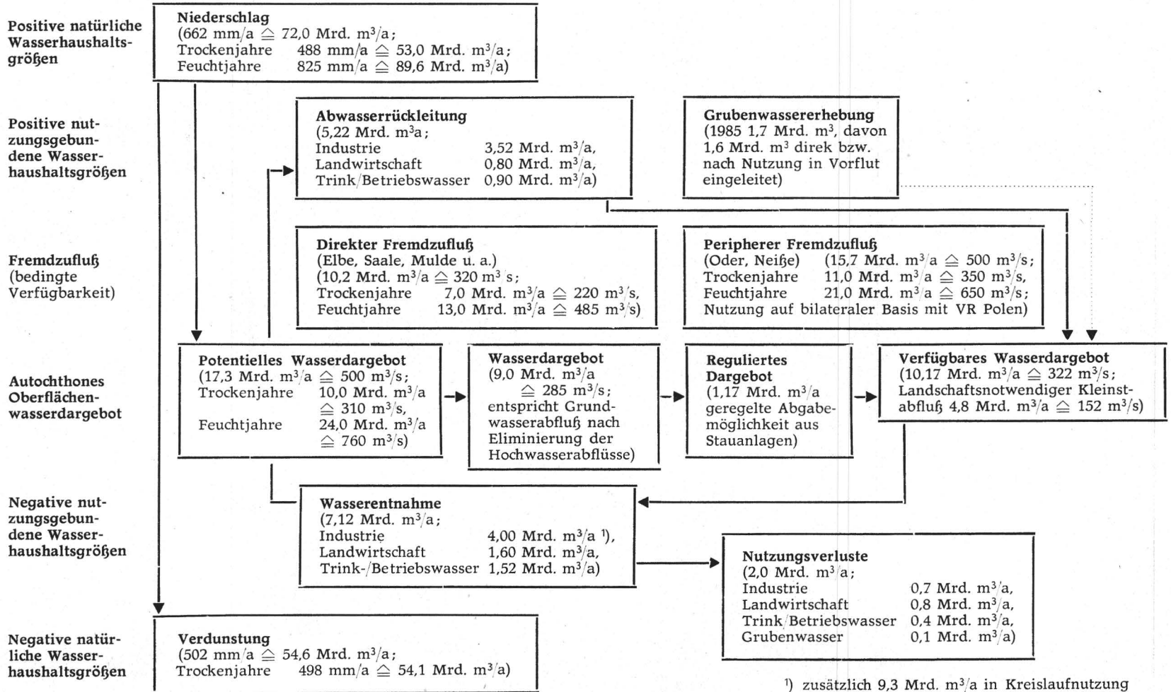
Abb. 1. Wasserhaushaltsschema der DDR (nach Dyck 1979/1982/1987 und Aurada 1983/1984/1986, ergänzt)
