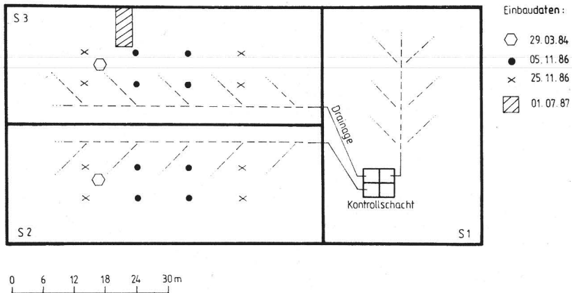
Abb. 1. Topographie der Versuchsdeponie mit Einbauorten und -zeitpunkten
