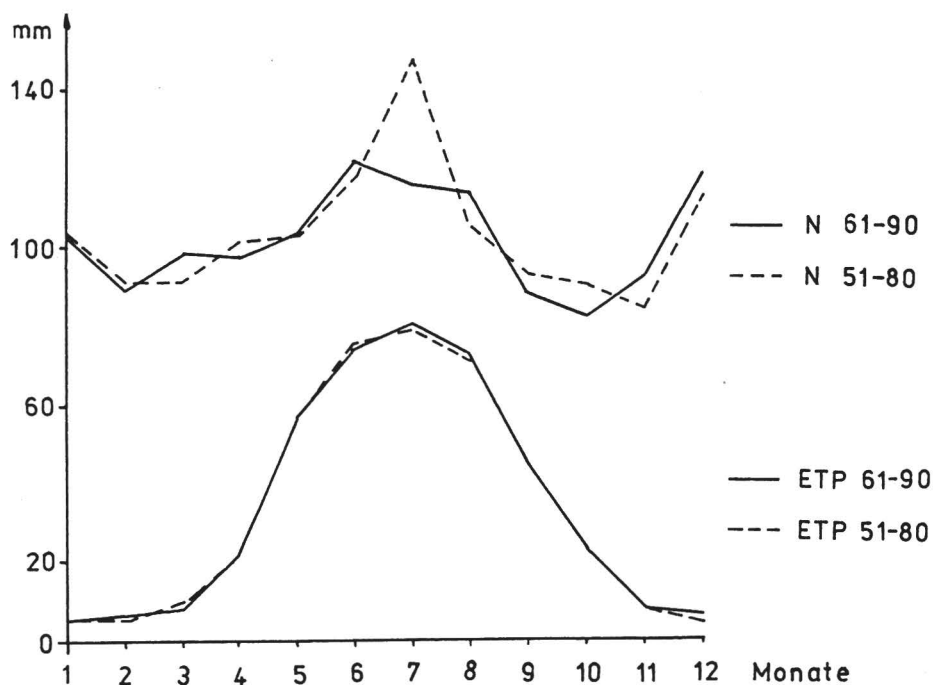
Abb. 6: Mittlere monatliche potentielle Verdunstung im Vergleich zu den Niederschlägen (Station Carlsfeld)
