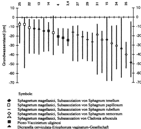
Abb. 1: Graphische Darstellung charakteristischer Grundwassermeßwerte: Gesamtamplitude und Medianwert (Symbol). Zu Meßstellen-Nummern und exakten Werten s. Tab. 7 (x-Achse = Meßstellen-Nummern).
