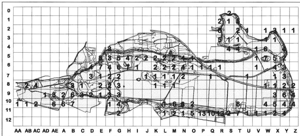
Abb. 3: Aktuelle Verbreitung ausgewählter Salzarten im Becken des Salzigen Sees (aktualisiert nach RANA 1998).
