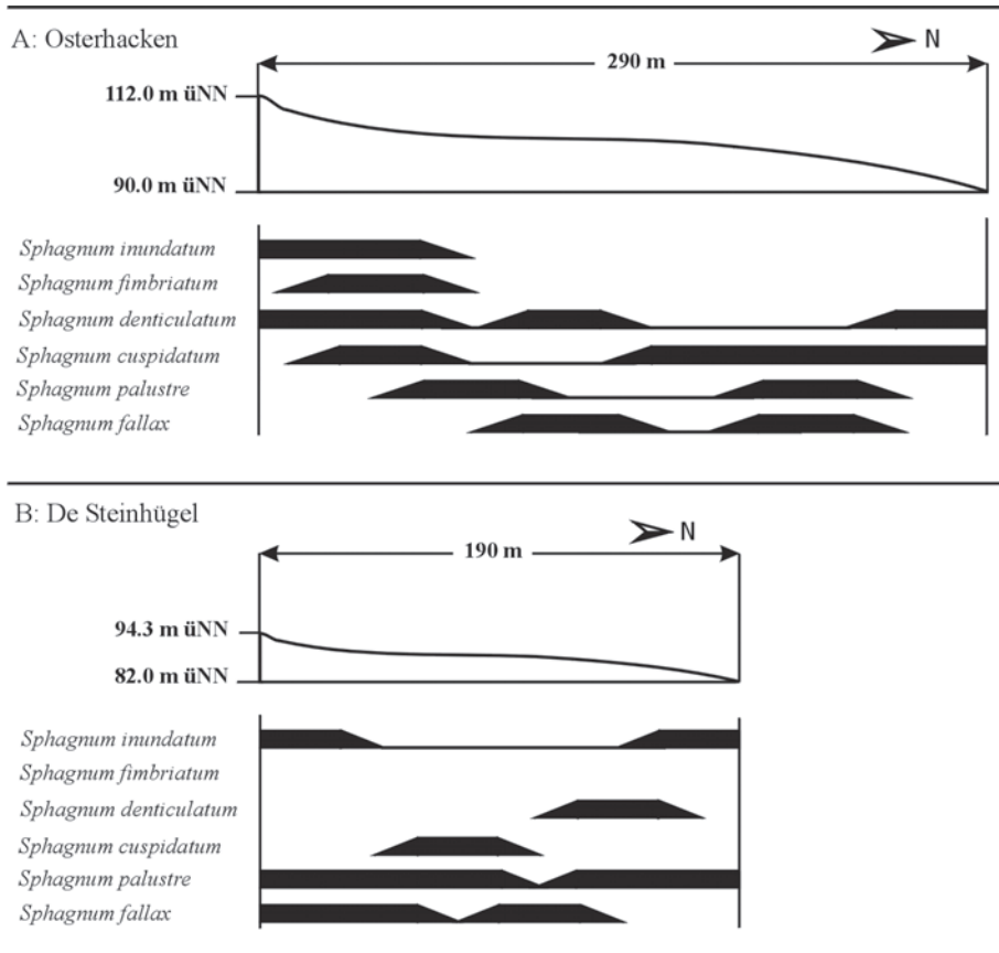
Abb. 2: Schematisches Artenprofil der Torfmoose ( Sphagnum spp.) aus Transexterfassungen entlang des Reliefgradienten in zwei Quellfluren am Riesenbecker Osning/ Nordwestlicher Teutoburger Wald (A: Osterhacken; B: De Steinhügel)
