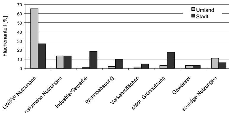
Abb. 3: Landschaftsstruktur der Untersuchungsgebiete – prozentuale Flächenanteile der Nutzungstypen (gruppiert). LW/FW Nutzungen = land- und forstwirtschaftliche Nutzungen, naturnahe Nutzungen = Staudenflur, naturnahes Gebüsch, Röhricht, Streuobstwiese, Wald
