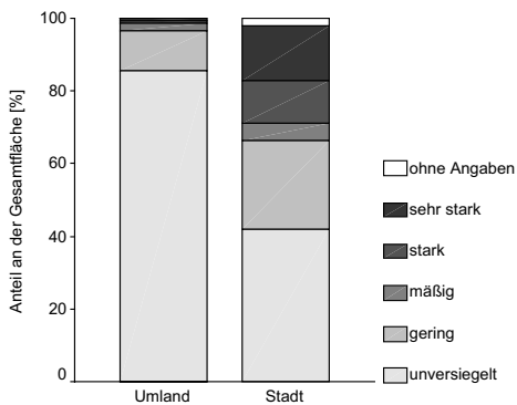
Abb. 4: Prozentuale Flächenanteile der Versiegelungsstufen an der Gesamtfläche der jeweils 20 Untersuchungsflächen in beiden Untersuchungsgebieten (p-Niveau Mann-Whitney U-Test: unversiegelt < 0,001 ; gering = 0,01; mäßig = 0,03; stark = 0,17; sehr stark = 0,01)
