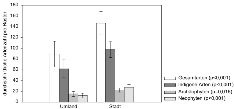
Abb. 2: Durchschnittliche Artenzahlen pro Raster (Fehlerbalken geben das 95 % Konfidenzintervall an) (p-Niveau Mann-Whitney U-Test)
