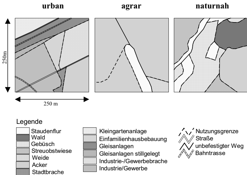
Abb. 6: Einfluß der Flächennutzung auf die Strukturvielfalt, dargestellt am Beispiel von drei unterschiedlich geprägten Untersuchungsflächen
