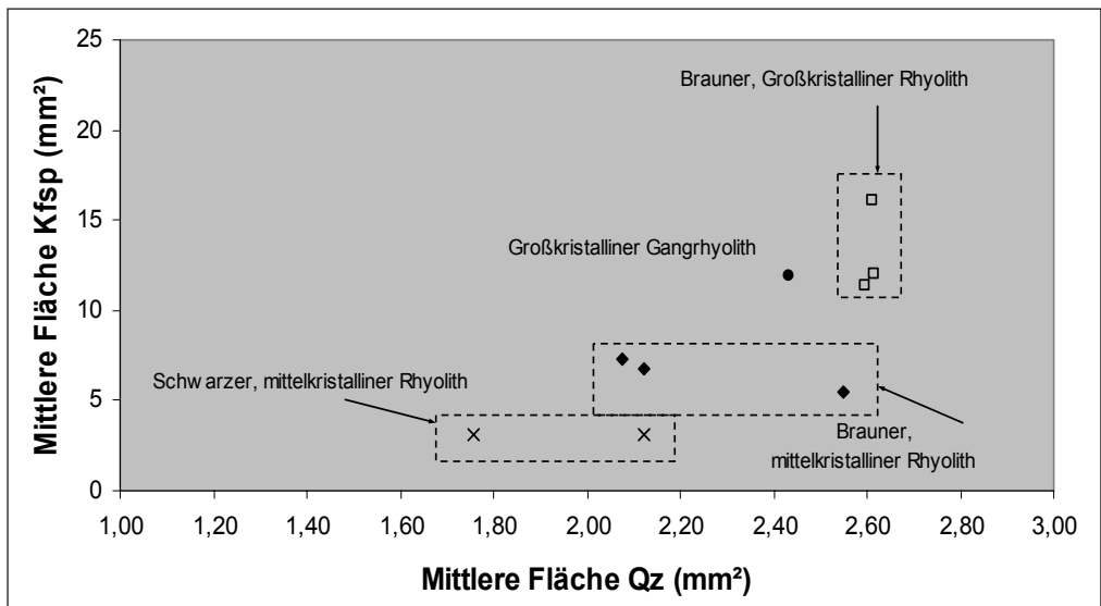
Abb. 14 Vergleich der verschiedenen Einheiten des Rhyolithkomplexes Scherz anhand des Verhältnisses der mittleren Fläche [mm 2 ] von Quarz (Qz) zu Kalifeldspat (Kfsp)
