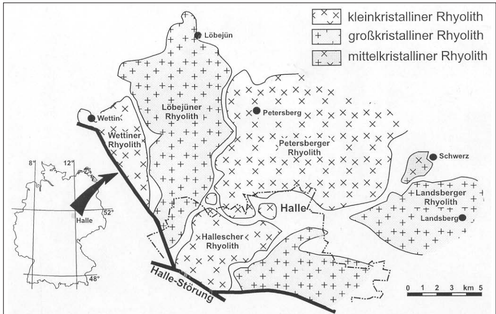
Abb. 6 Übersichtskarte des Halleschen Vulkanitkomplexes (EXNER et SCHWAB 2000)
