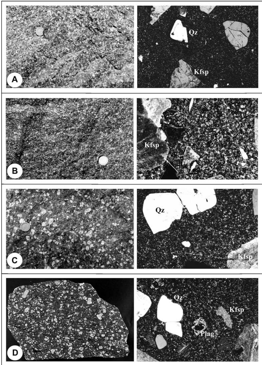
Abb. 10 Rhyolithvarietäten Schwerz (links: Anschliffe, rechts: Dünnschliffe)
