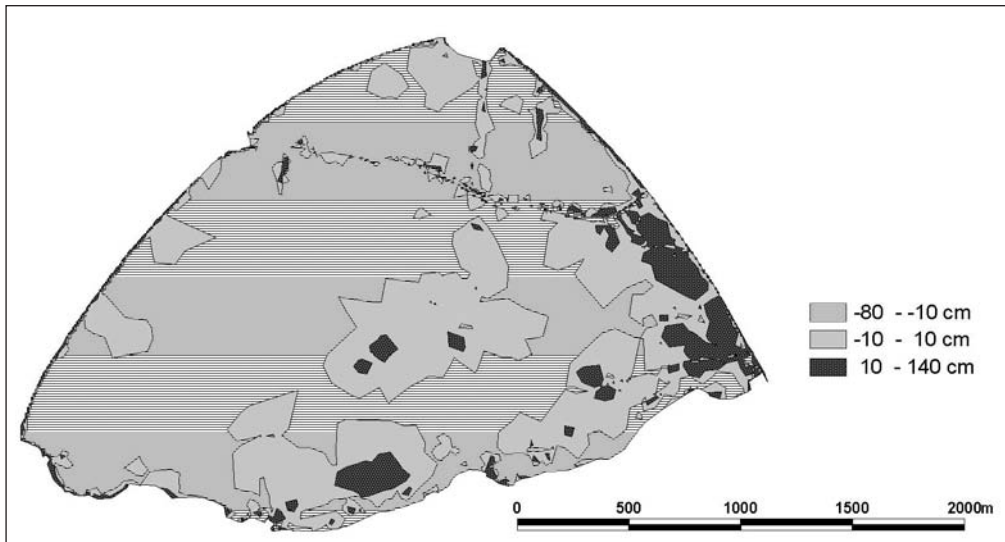
Abb. 6 Höheniveauänderung 1994–2001
