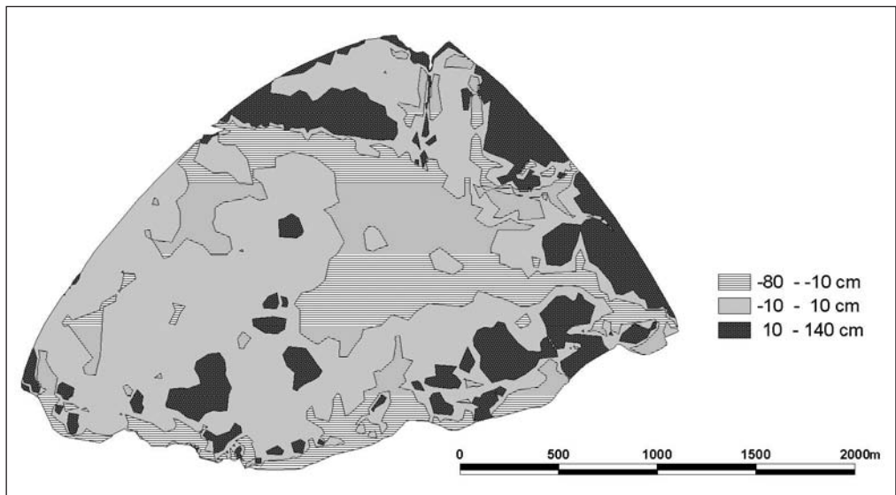
Abb. 5 Höhenniveaünderung 1952–1994
