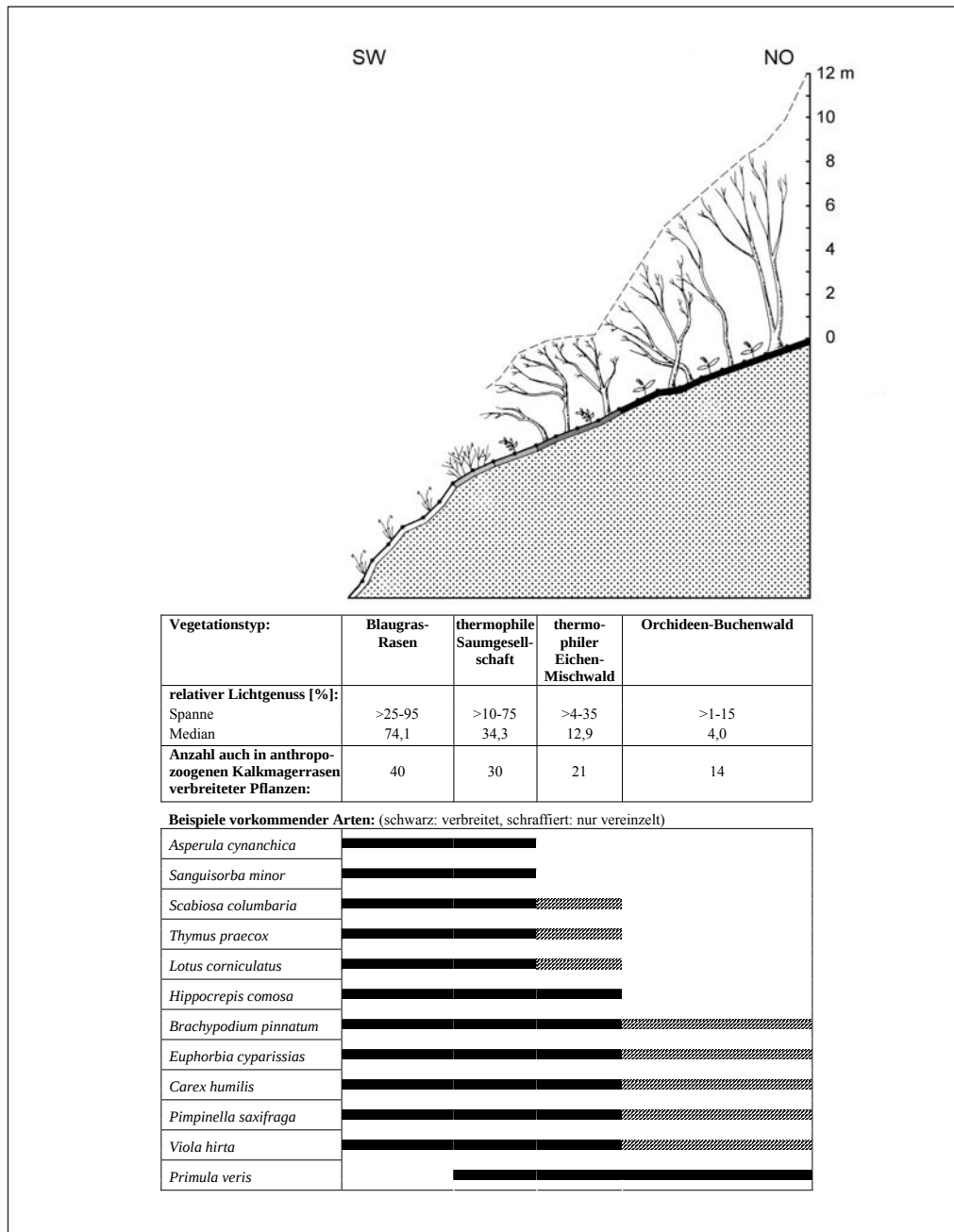
Abb. 3 Vegetationsabfolge eines trockenheitsbedingten Waldgrenzstandortes im nördlichen deutschen Hügelland nach SCHMIDT (2000). Weitere Angaben zu den Lichtansprüchen der Vegetationstypen und Pflanzenarten siehe dort.
