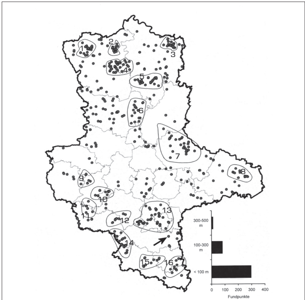
Abb. 2 Verbreitungsschwerpunkte (VSP) 1–16 und Höhenverbreitung des Kammolchs in Sachsen-Anhalt, Schwarzer Pfeil – Vorkommen Untersuchungsgebiet Merseburg
